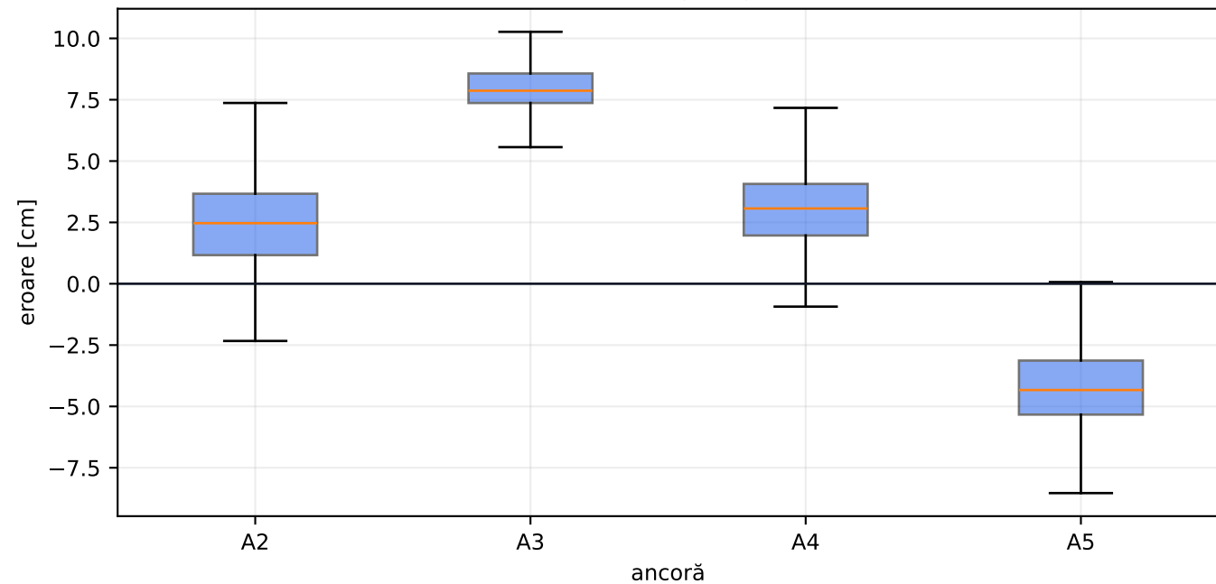
DS-TWR: eroarea distanței față de 2,12132 m
