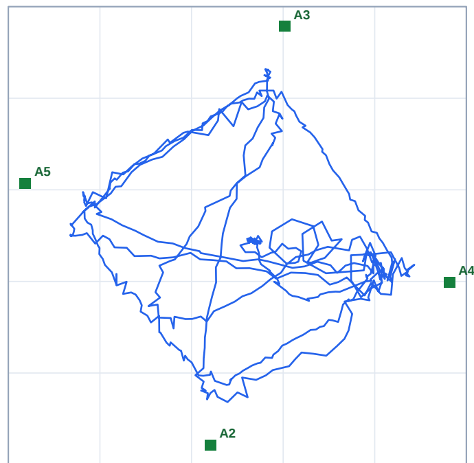
Native DS-TWR
