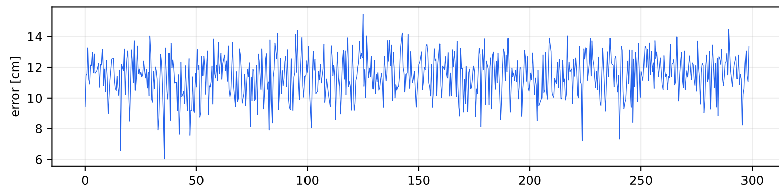
Passive DS-TWR
