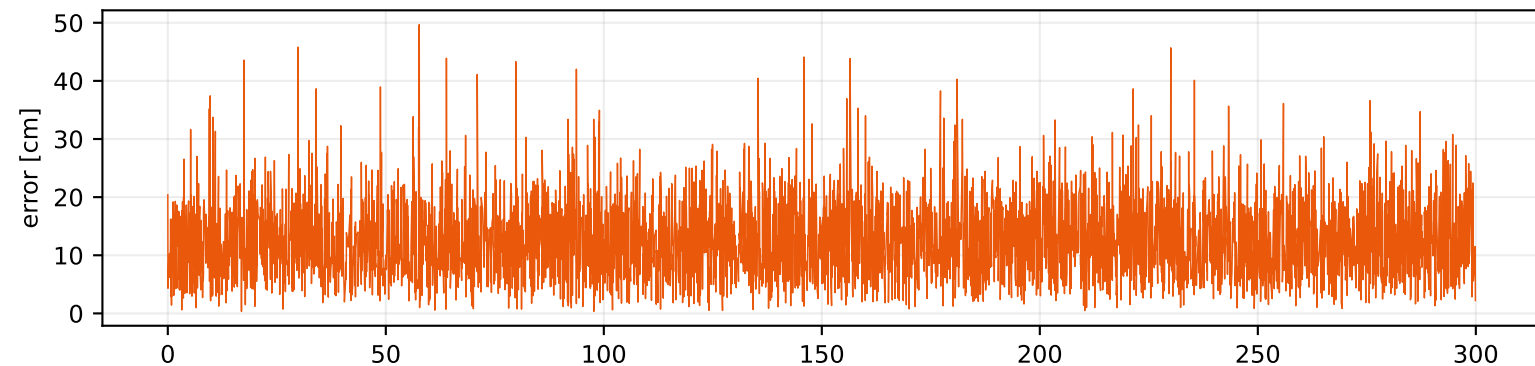
Native DS-TWR
