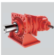
JRP Redutores planetários Tamanho: 9–36 Relação: 25–4000 Potência de entrada: 0,4–12,934 kW Torque de saída: 22000–2600000 N·m
