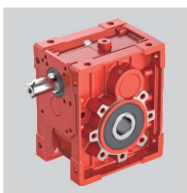
JBKM Redutores hipoidais Tamanho: 28–68 Relação: 7,5–300 Potência de entrada: 0,07–11,1 kW Torque de saída: 12–886 N·m
