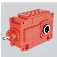
JRHB Redutores cônicos helicoidais Tamanho: 4–28 Relação: 5–400 Potência de entrada: 2,8–4908 kW Torque de saída: 5500–1400000 N·m
