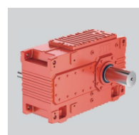
JRTH Motorreduztor helicoidal com rosca sem-fim Tamanho: 39–99 Relação: 6,8–288 Potência de entrada: 0,12–22 kW Torque de saída: 10–4900 N·m
