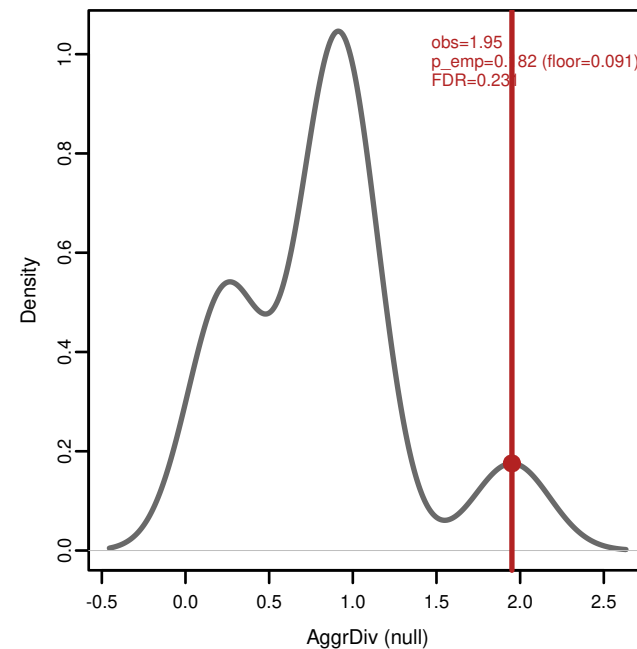
T4 (n=3 v 2, pool=5)
