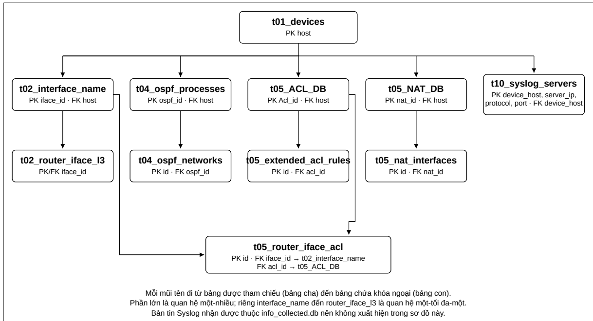
Hình 3.6: Lược đồ khóa ngoại đại diện trong cơ sở dữ liệu device_network.db
