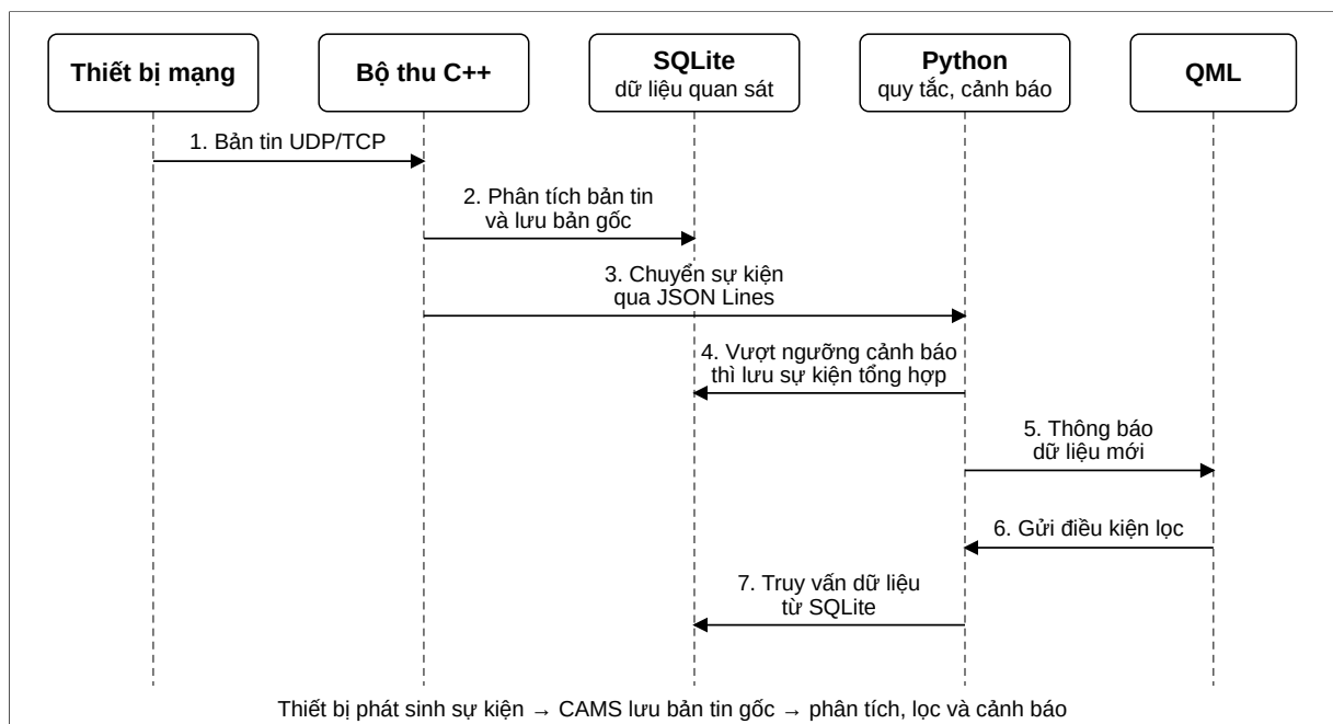
Hình 3.5: Sơ đồ tuần tự thu nhận, lưu trữ và khai thác Syslog
