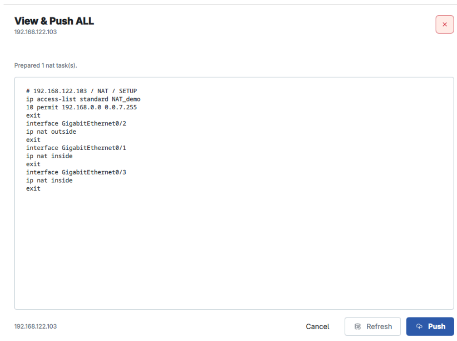
Hình 5.21: Cửa sổ View & Push sinh cấu hình cổng NAT và ACL cho bộ định tuyến NAT
