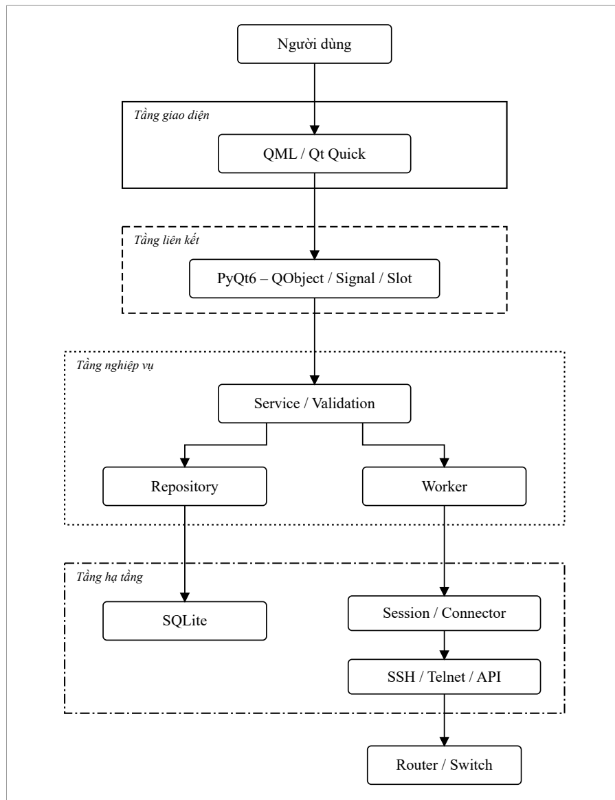
Hình 3.2: Kiến trúc phân lớp của CAMS
