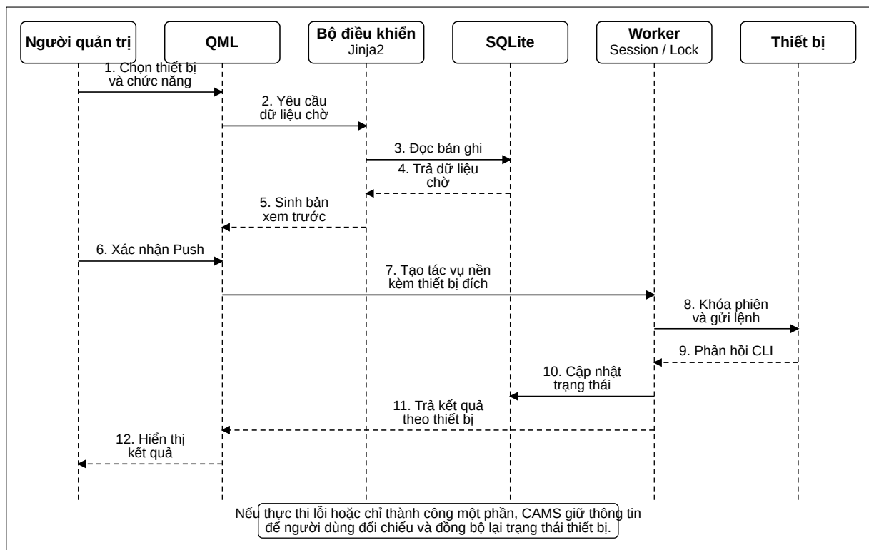
Hình 3.4: Sơ đồ tuần tự của quy trình View & Push
