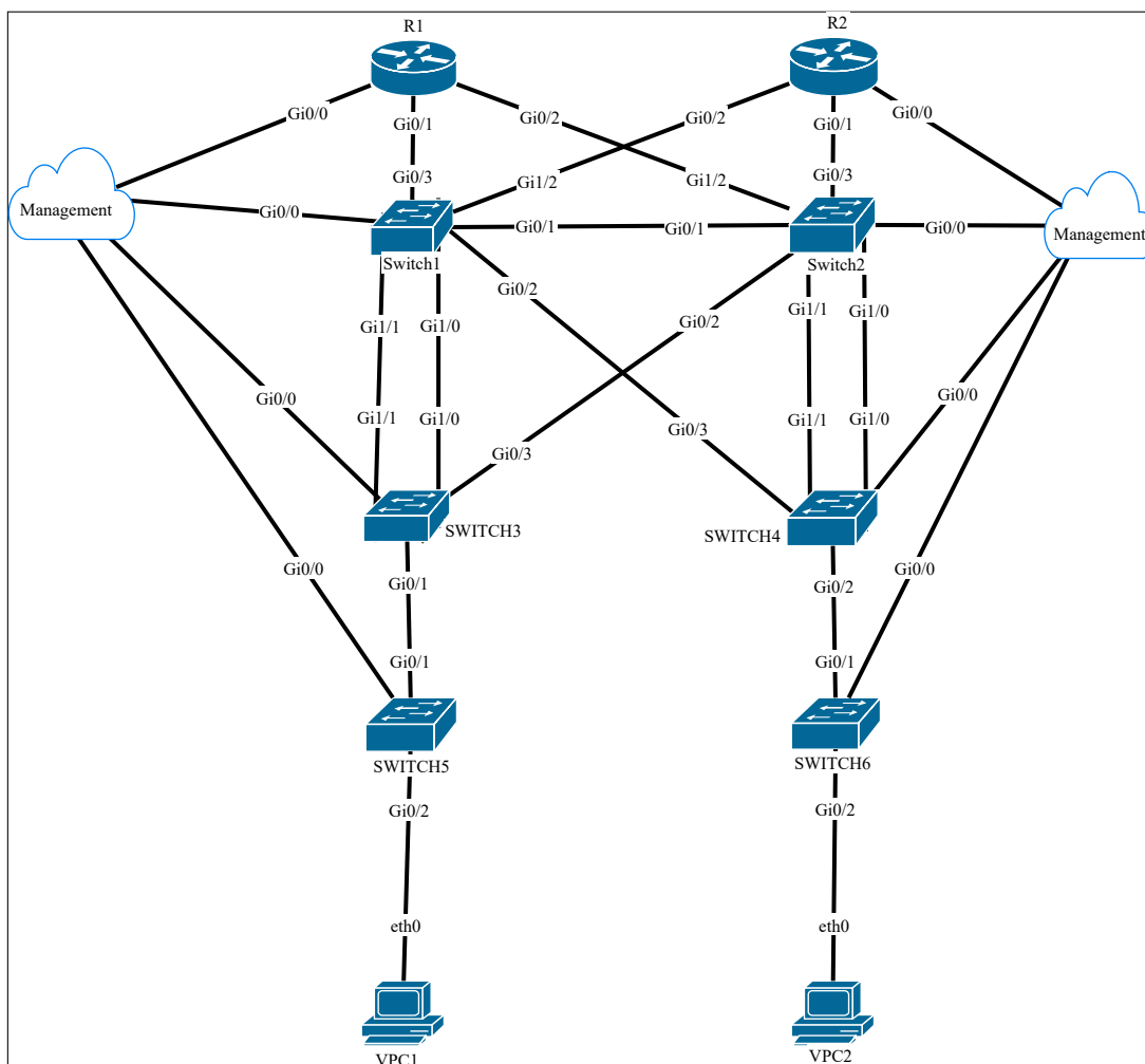
Hình 5.1: Sơ đồ Topo Kịch bản 1: Hạ tầng Chuyển mạch và Bảo mật Lớp 2
