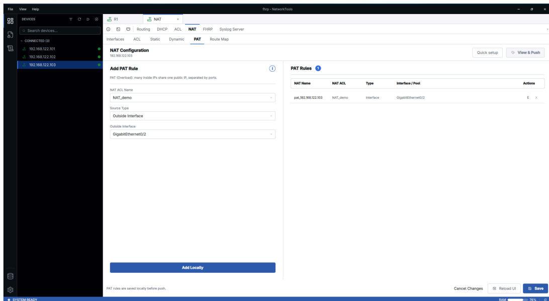
Hình 5.28: Giao diện cấu hình PAT Overload sử dụng cổng Outside GigabitEthernet0/2
