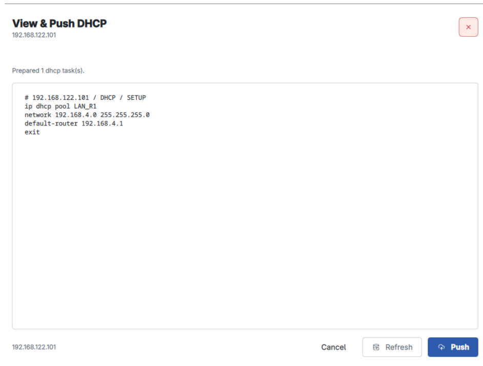
Hình 5.36: Cửa sổ View & Push DHCP sinh cấu hình pool LAN_R1 trên R1
