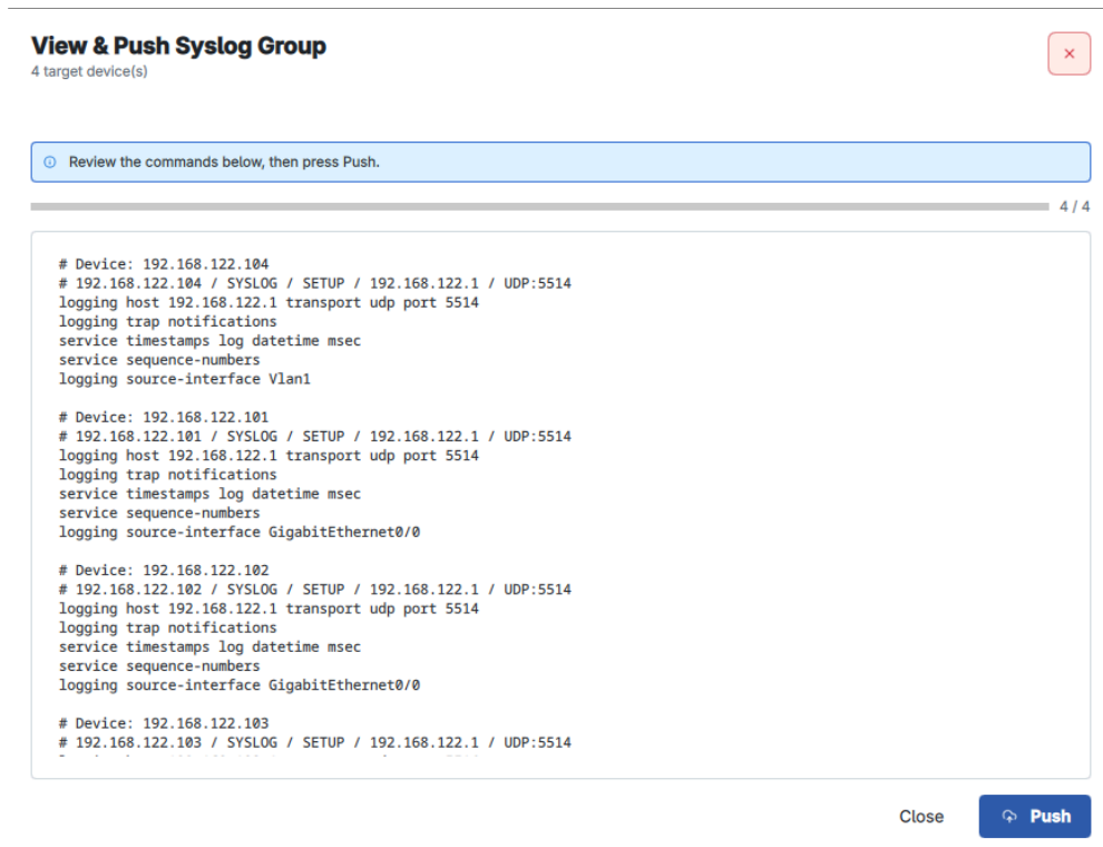
Hình 5.45: Cửa sổ View & Push Syslog Group tổng hợp lệnh cho 4 thiết bị trước khi thực thi
