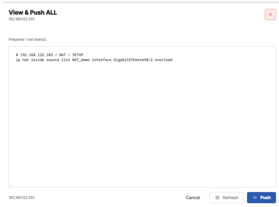
Hình 5.29: Cửa sổ View & Push kiểm duyệt lệnh PAT Overload trước khi đẩy xuống Router NAT
