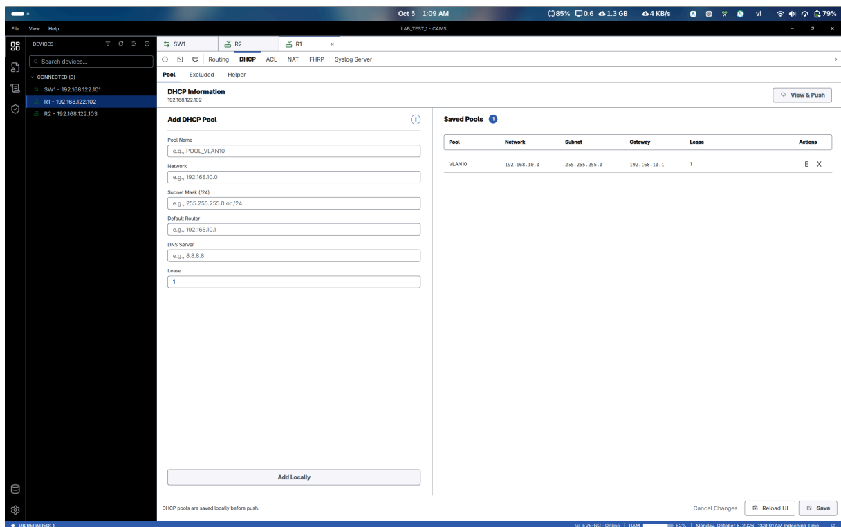
Hình 5.3: Pool DHCP trên R1 dùng làm nguồn cấp phát ở trạng thái A.
