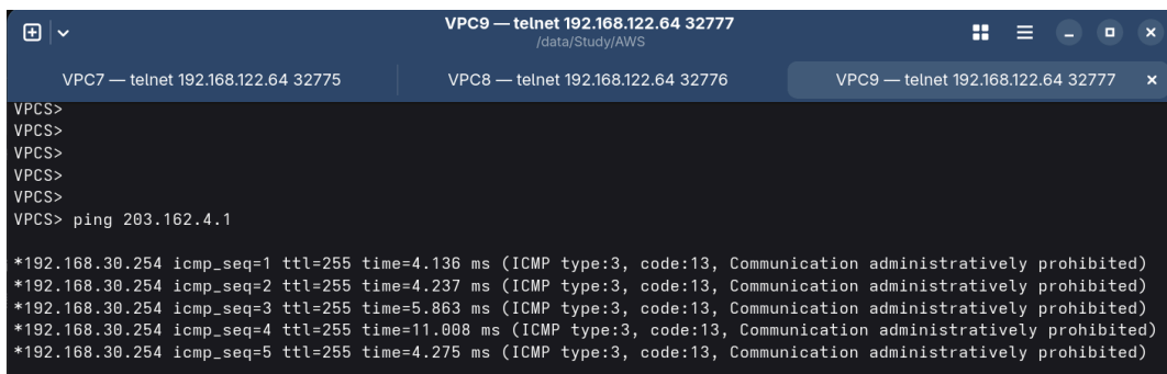
Hình 5.64: R1 từ chối ICMP từ VLAN 30 đến máy chủ 203.162.4.1
