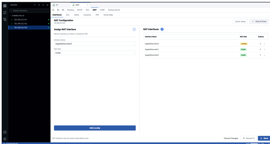
Hình 5.25: Giao diện cấu hình cổng NAT Inside/Outside trên Router NAT
