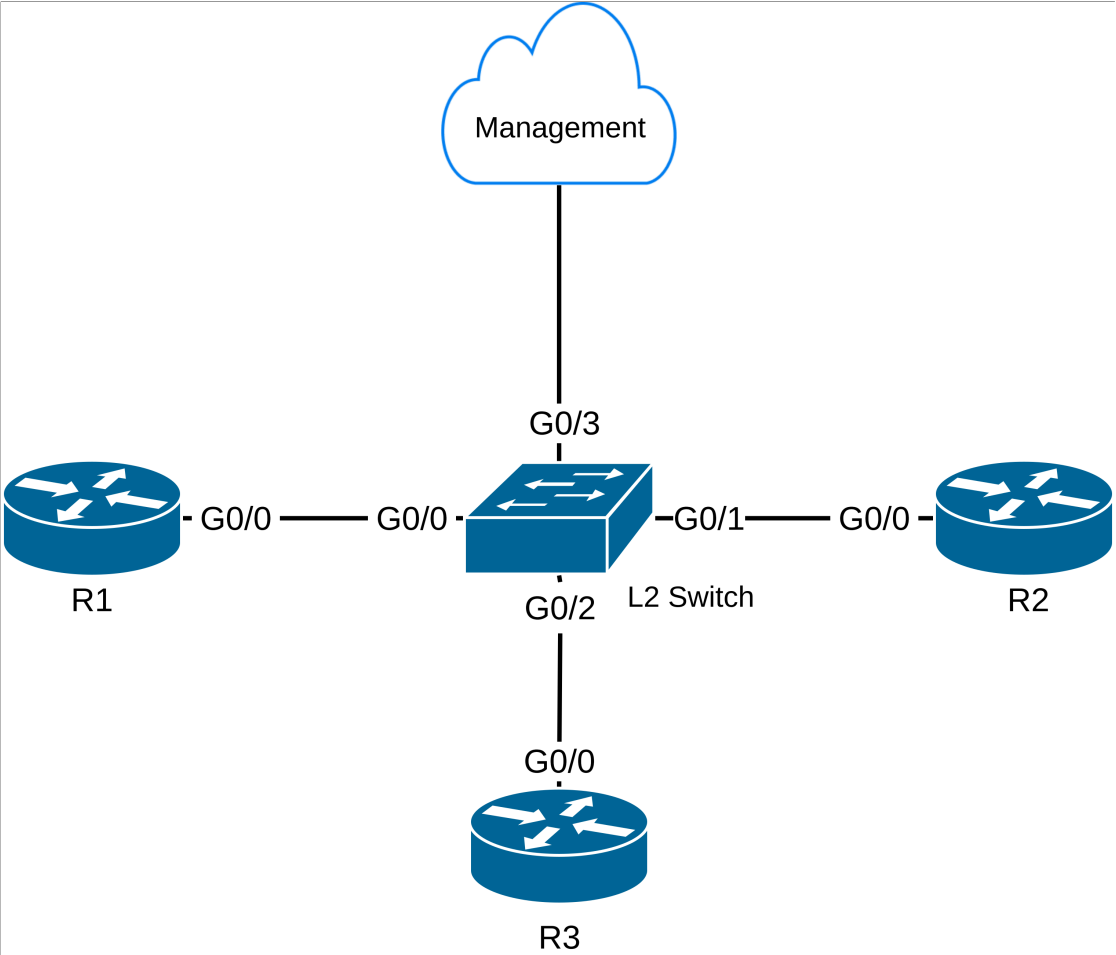
Hình 5.40: Sơ đồ Kịch bản 4: Thu thập Syslog tập trung
