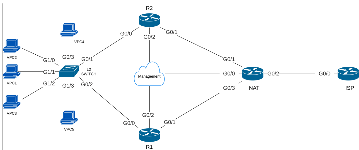
Hình 5.24: Sơ đồ Kịch bản 2: Tích hợp GLBP, DHCP và NAT/PAT cho mạng LAN
