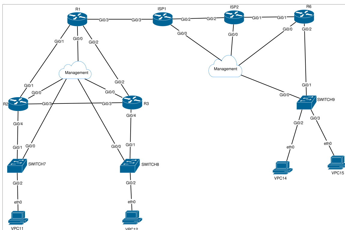
Hình 5.15: Sơ đồ Kịch bản 1: Định tuyến OSPF đa vùng giữa hai chi nhánh
