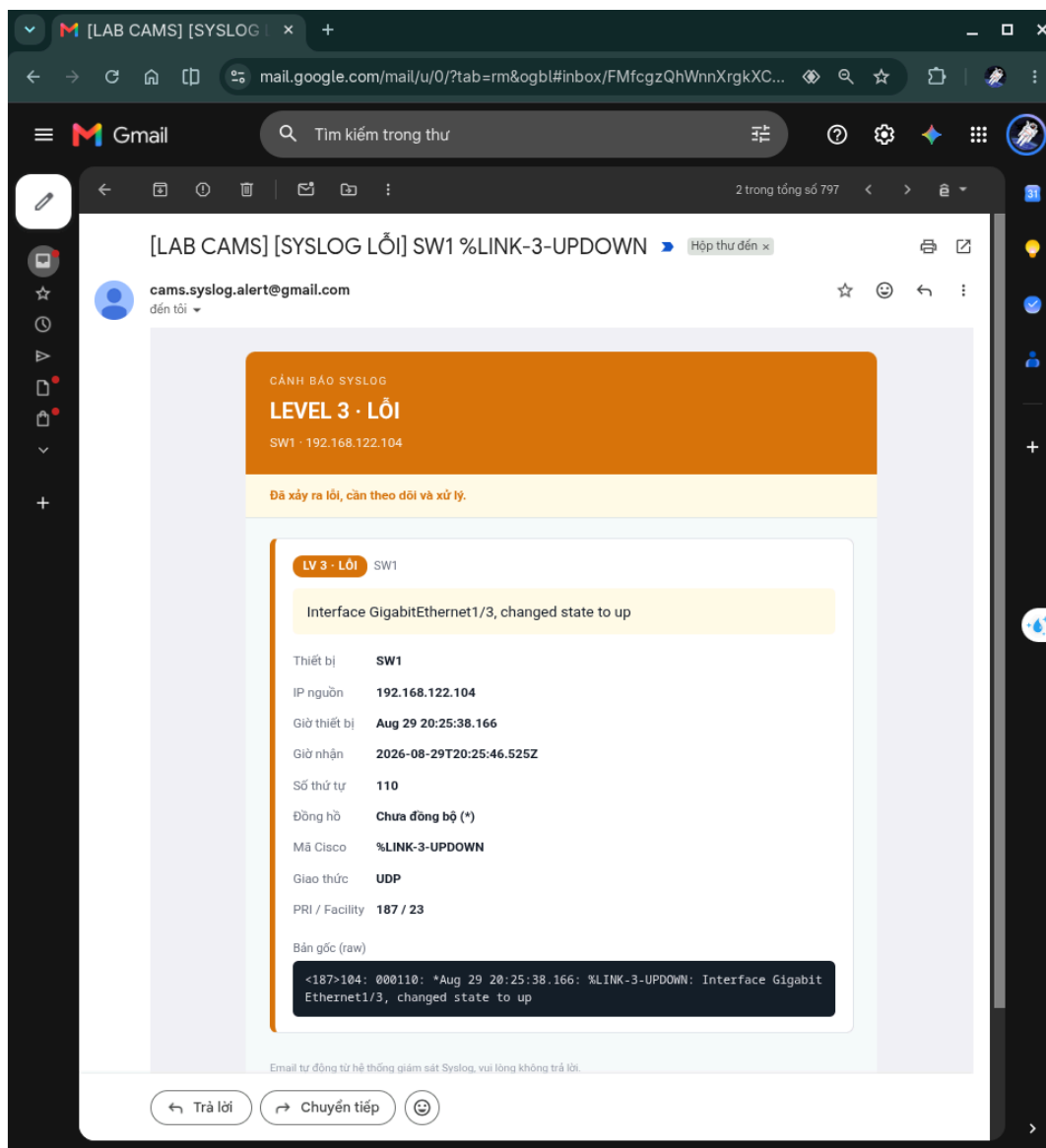
Hình 5.54: Minh họa email cảnh báo mức Error cho sự kiện %LINK-3-UPDOWN trên SW1
