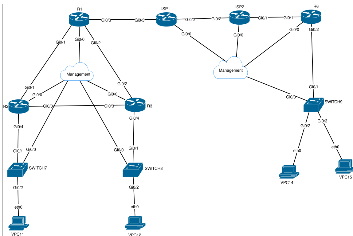
Hình 5.11: Sơ đồ Kịch bản 1: Định tuyến OSPF đa vùng giữa hai chi nhánh
