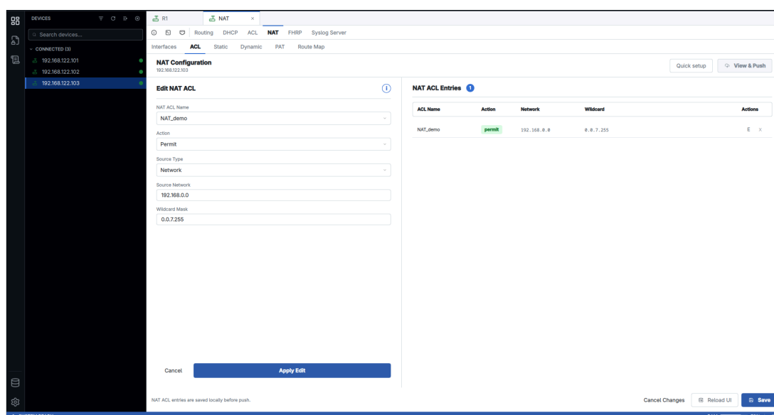
Hình 5.22: Khai báo ACL NAT_demo xác định các mạng nội bộ được phép chuyển đổi địa chỉ
