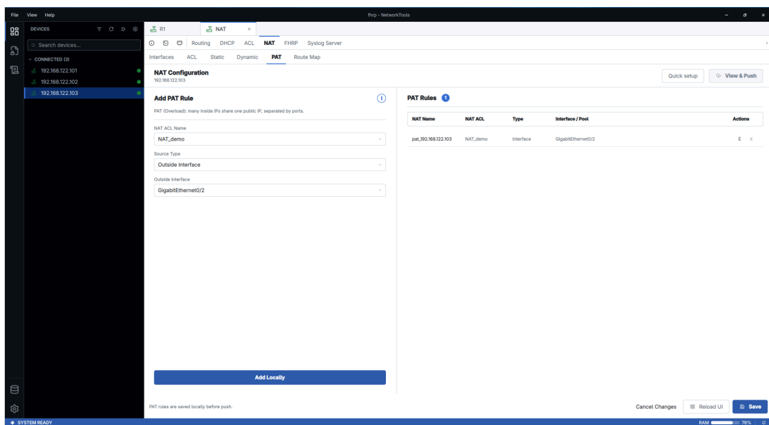
Hình 5.24: Giao diện cấu hình PAT Overload sử dụng cổng Outside GigabitEthernet0/2
