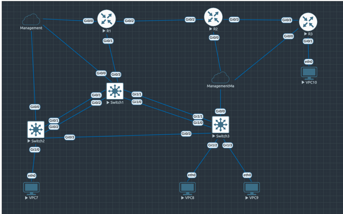
Hình 5.56: Mô hình kiểm chứng ACL với R1 định tuyến liên VLAN, R2 làm NAT và R3 làm ISP
