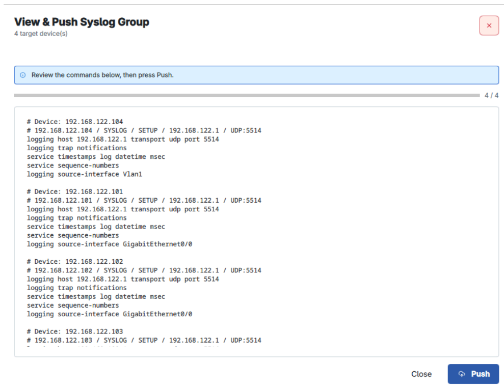
Hình 5.41: Cửa sổ View & Push Syslog Group tổng hợp lệnh cho 4 thiết bị trước khi thực thi
