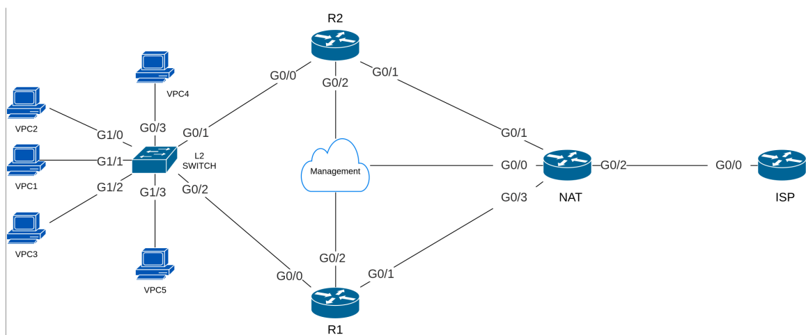
Hình 5.20: Sơ đồ Kịch bản 2: Tích hợp GLBP, DHCP và NAT/PAT cho mạng LAN
