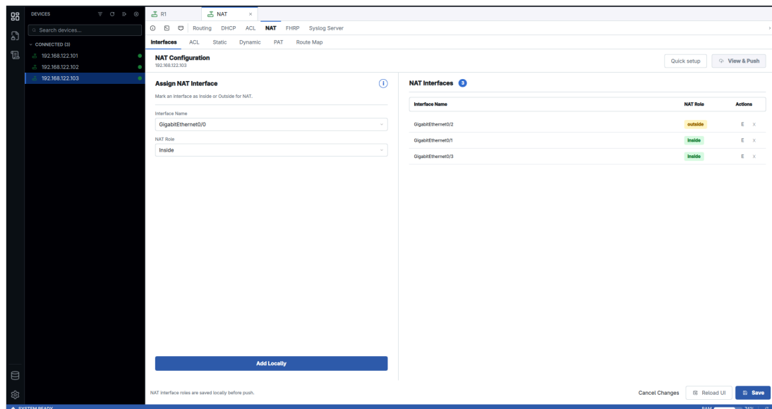
Hình 5.21: Giao diện cấu hình cổng NAT Inside/Outside trên Router NAT
