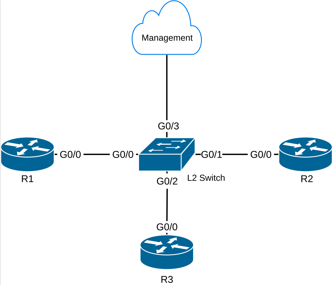
Hình 5.36: Sơ đồ Kịch bản 4: Thu thập Syslog tập trung
