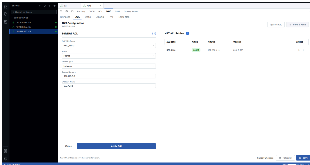
Hình 5.19: Khai báo ACL NAT_demo xác định các mạng nội bộ được phép chuyển đổi địa chỉ
