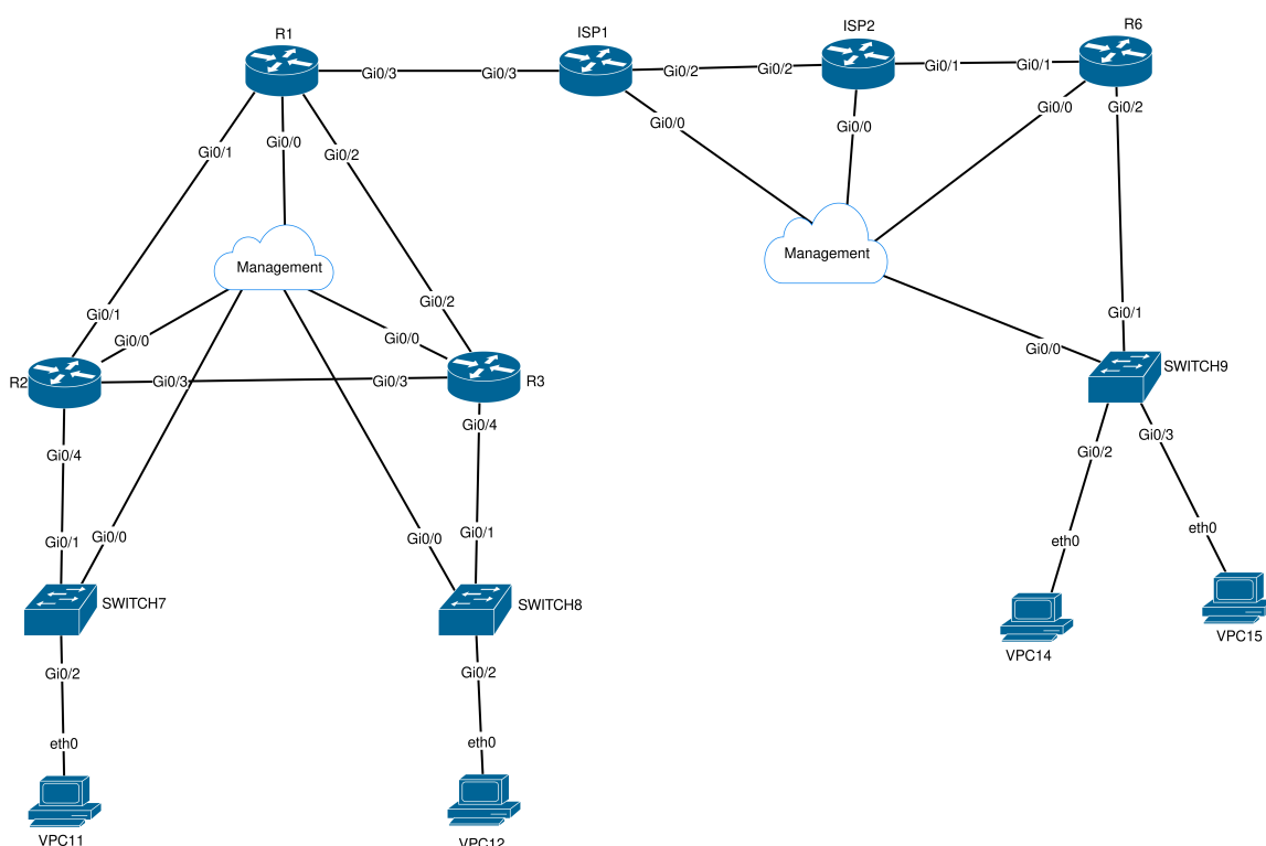
Hình 5.1: Sơ đồ Topo Kịch bản 1: Định tuyến OSPF đa vùng giữa hai chi nhánh
