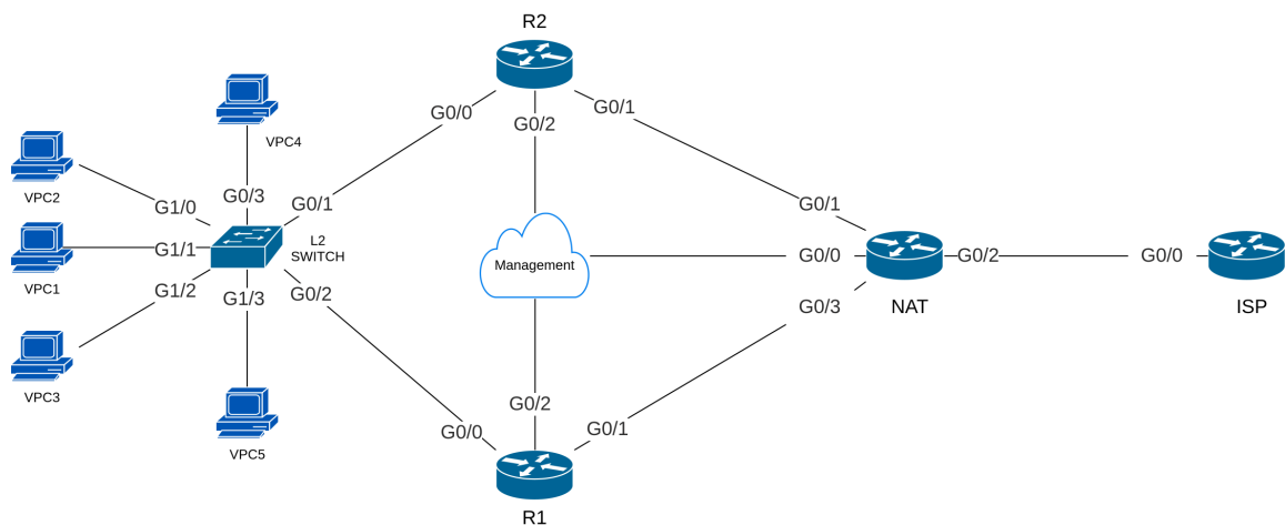
Hình 5.10: Sơ đồ Topo Kịch bản 2: Tích hợp GLBP, DHCP và NAT/PAT cho mạng LAN
