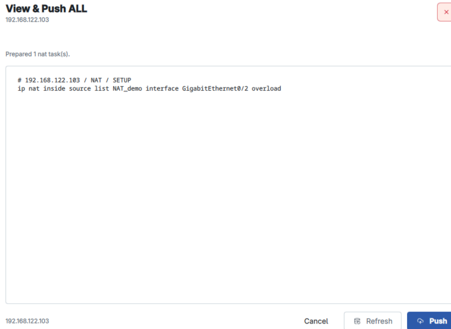
Hình 5.15: Cửa sổ View & Push kiểm duyệt lệnh PAT Overload trước khi đẩy xuống Router NAT
