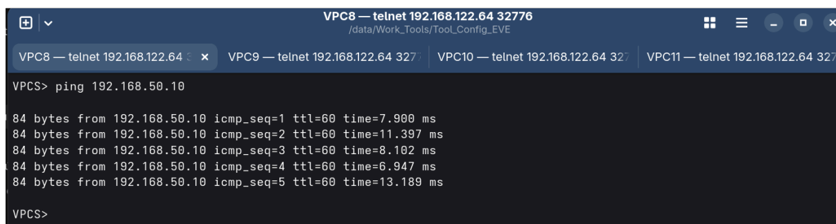
Hình 5.17: VPC8 nhận đủ năm hồi đáp ICMP từ VPC10 ở LAN phía sau R5
