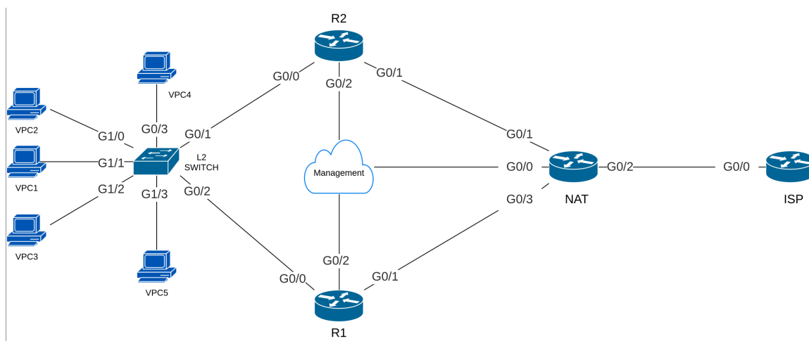
Hình 5.18: Sơ đồ Kích bản 3: Tích hợp GLBP, DHCP và NAT/PAT cho mạng LAN
