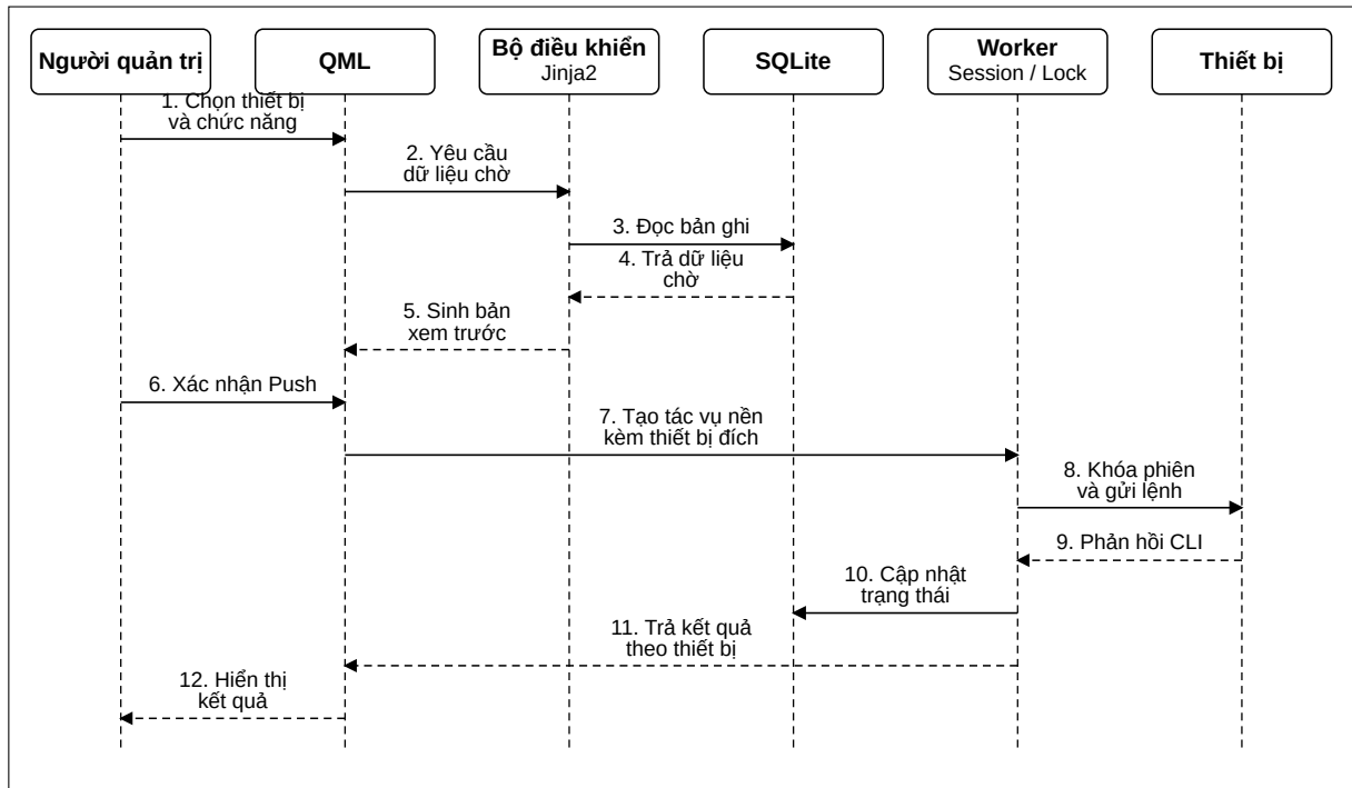
Hình 3.3: Sơ đồ tuần tự của quy trình View & Push
