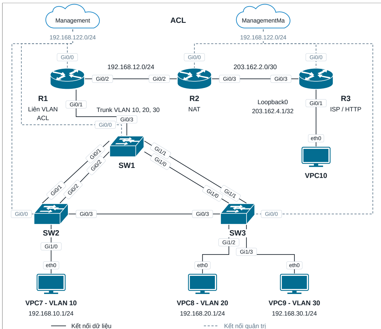
Hình 5.54: Mô hình kiểm chứng ACL với R1 định tuyến liên VLAN, R2 làm NAT và R3 làm ISP (vẽ lại từ topology EVE-NG)
