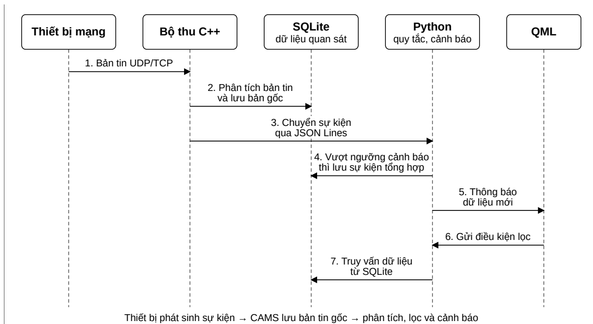
Hình 3.4: Sơ đồ tuần tự thu nhận, lưu trữ và khai thác Syslog
