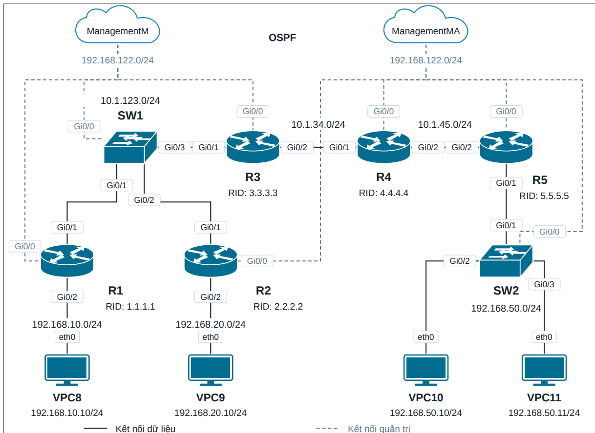
Hình 5.11: Mô hình thử nghiệm OSPF một vùng gồm năm bộ định tuyến, hai bộ chuyển mạch và bốn máy trạm (vẽ lại từ topology EVE-NG)
