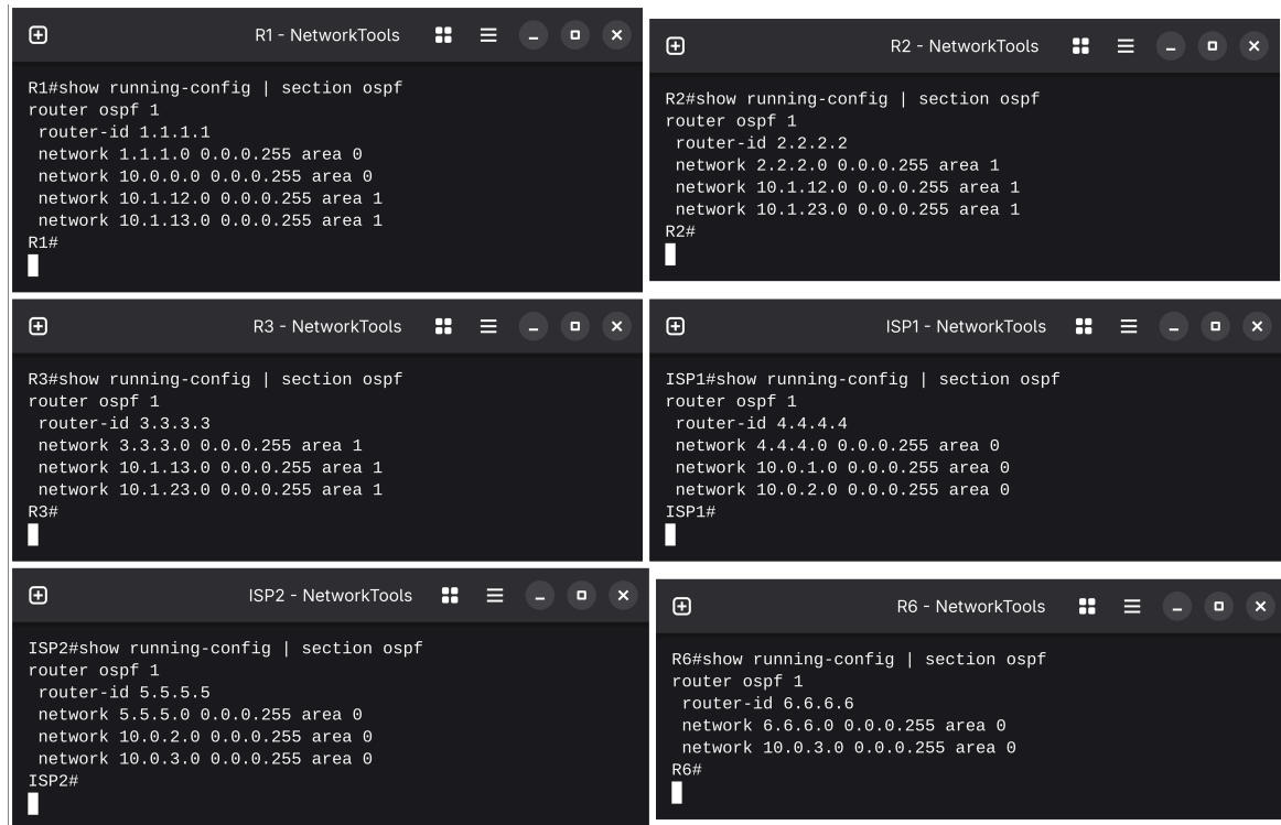
Hình 5.14: Xác minh cấu hình OSPF trên sáu router qua terminal nhúng
