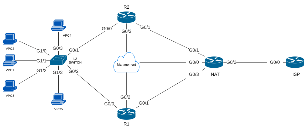
Hình 5.17: Sơ đồ Kịch bản 2: Tích hợp GLBP, DHCP và NAT/PAT cho mạng LAN
