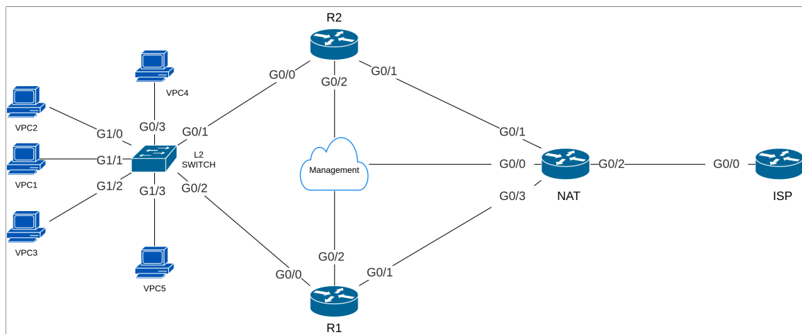
Hình 5.18: Sơ đồ Kịch bản 3: Tích hợp GLBP, DHCP và NAT/PAT cho mạng LAN
