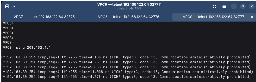
Hình 5.57: R1 từ chối ICMP từ VLAN 30 đến máy chủ 203.162.4.1
