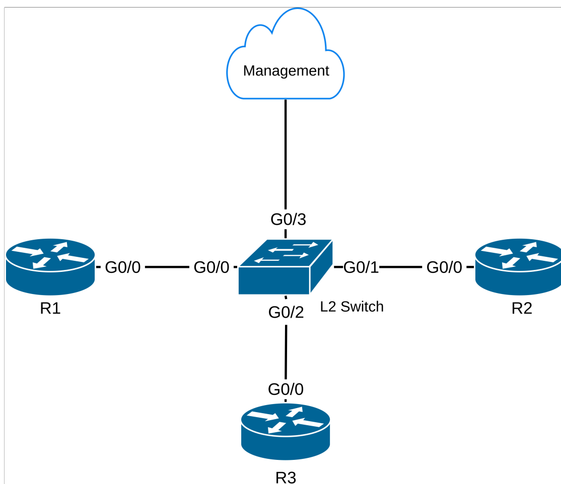
Hình 5.33: Sơ đồ Kịch bản 4: Thu thập Syslog tập trung
