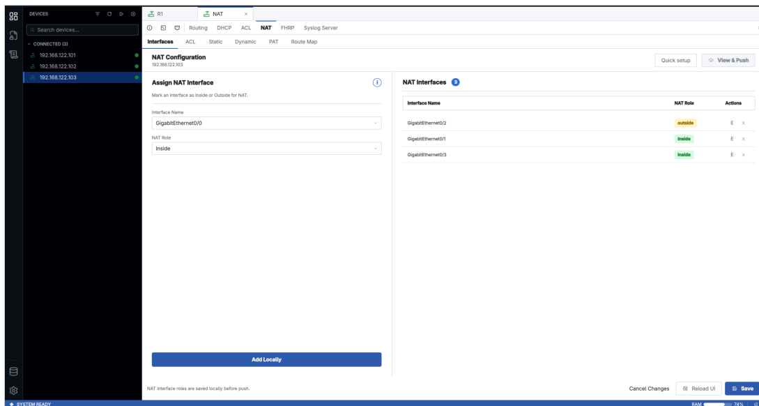
Hình 5.18: Giao diện cấu hình cổng NAT Inside/Outside trên Router NAT
