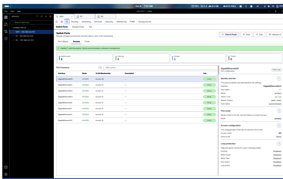
Hình 5.2: Giao diện CAMS cấu hình phân vùng VLAN 10 và các cổng Access trên SW1
