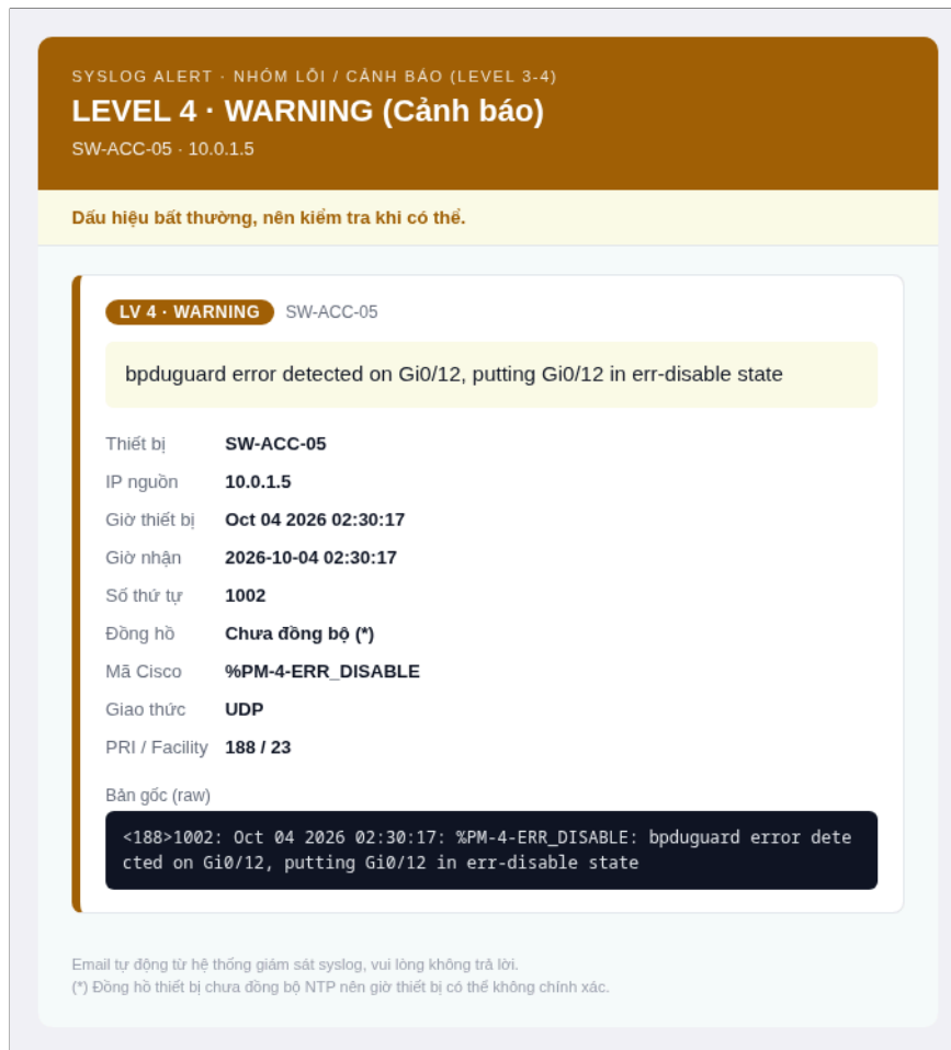
Hình 5.52: Email cảnh báo mức Warning cho sự kiện %PM-4-ERR_DISABLE
