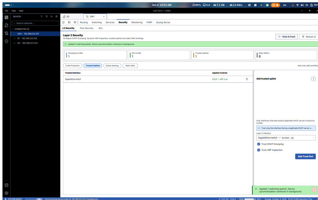
Hình 5.5: Chỉ định cổng GigabitEthernet0/1 làm Trusted Uplink cho DHCP Snooping trên CAMS
