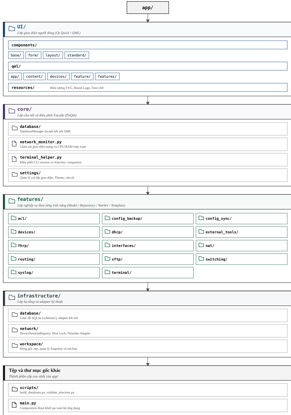
Hình A.1: Sơ đồ cấu trúc thư mục mã nguồn ứng dụng desktop CAMS (thư mục app/)
