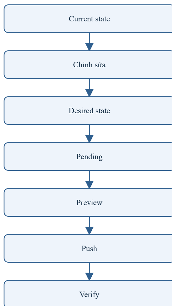
Hình 2.2: Vòng đời một thay đổi cấu hình theo trạng thái
