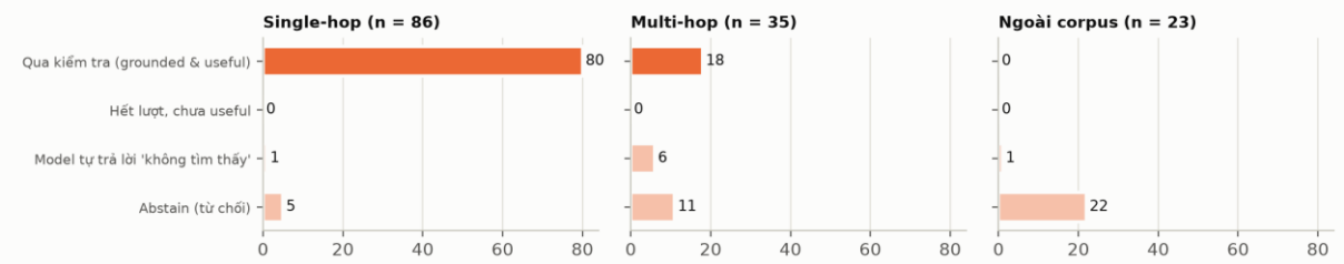
Hình 8. Trạng thái kết thúc của Self-RAG theo loại câu hỏi, top-k = 4
