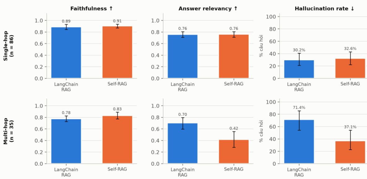
Hình 4. Ba chỉ số theo loại câu hỏi, top-k = 4
