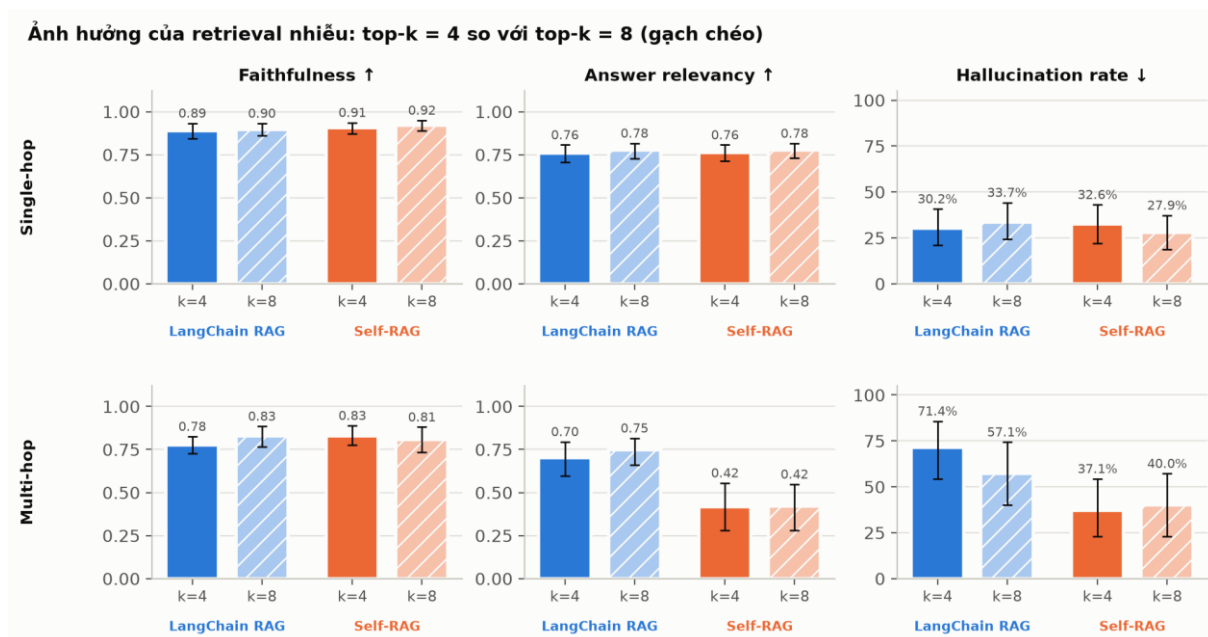
Hình 6. Ba chỉ số khi top-k = 4 và top-k = 8
