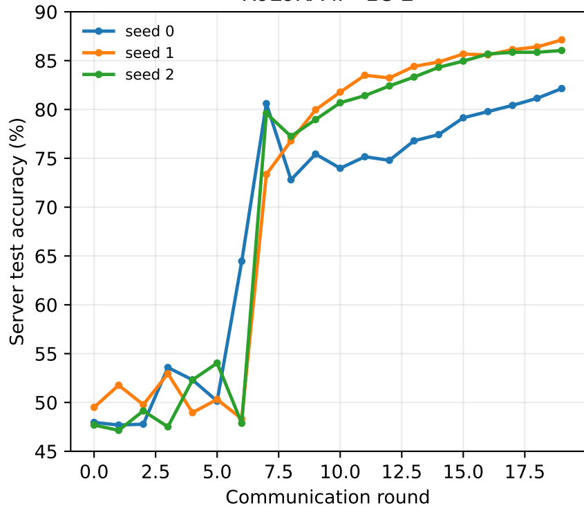
RoLoRA \text{lr}=1\text{e-}2
