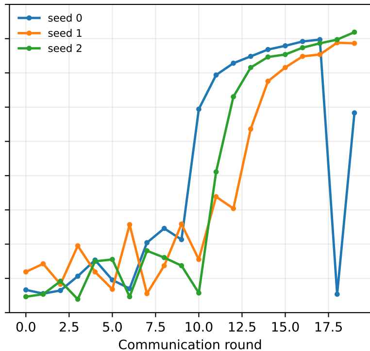
RoLoRA \text{lr}=5\text{e-}3
