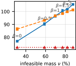
IMDb-Wiki: top identities (MSE)
