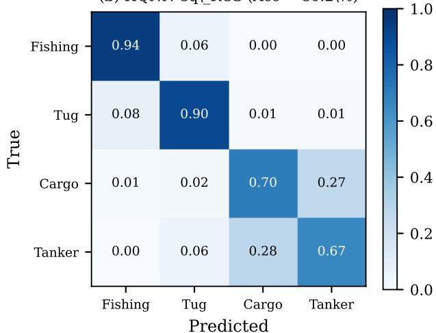
(b) HQNN-8q\RCS (Acc = 80.2\%)
