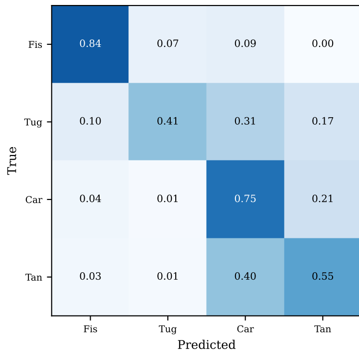
(d) Baseline OOF (67.7%)
