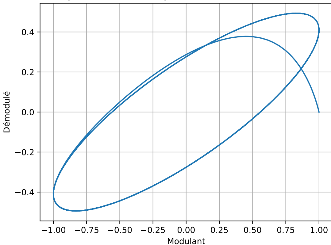
XY Plot du signal modulant vs signal démodulé (démodulation cohérente)
