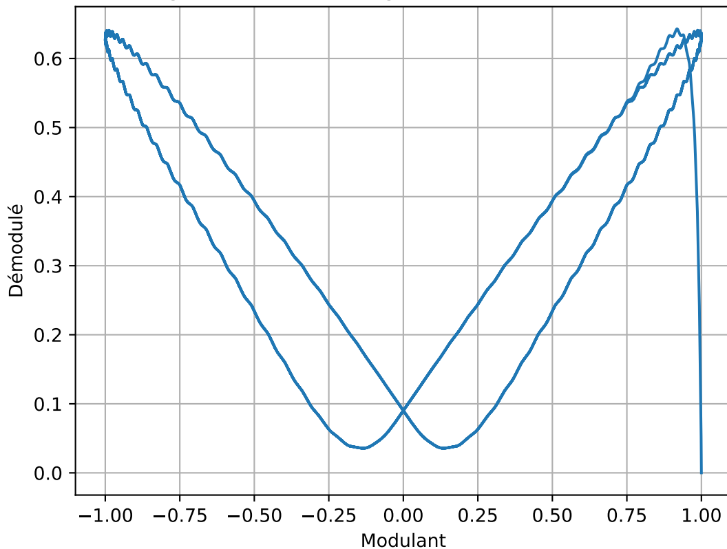
XY Plot du signal modulant vs signal démodulé (détecteur de crête)
