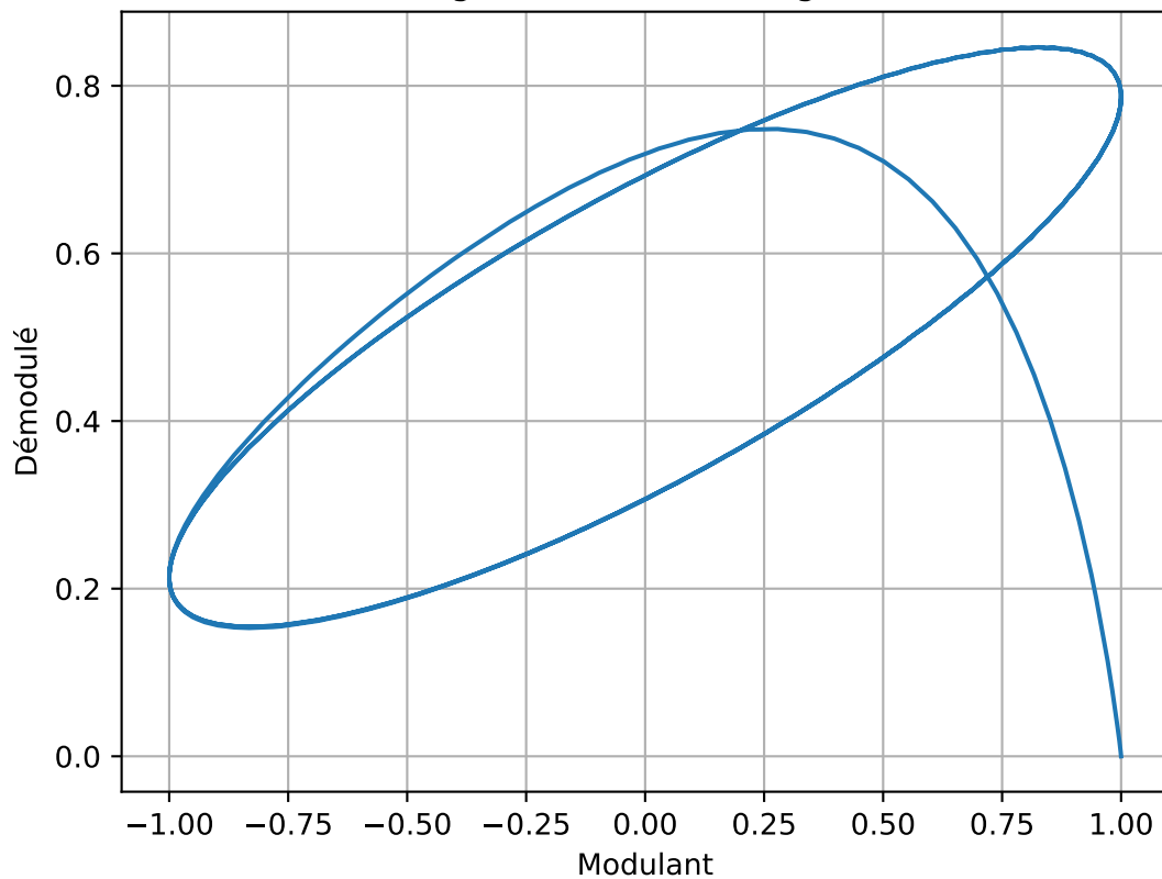
XY Plot du signal modulant vs signal démodulé
