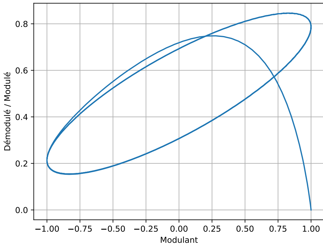
A3 — X-Y : modulant vs démodulé (cohérent)
