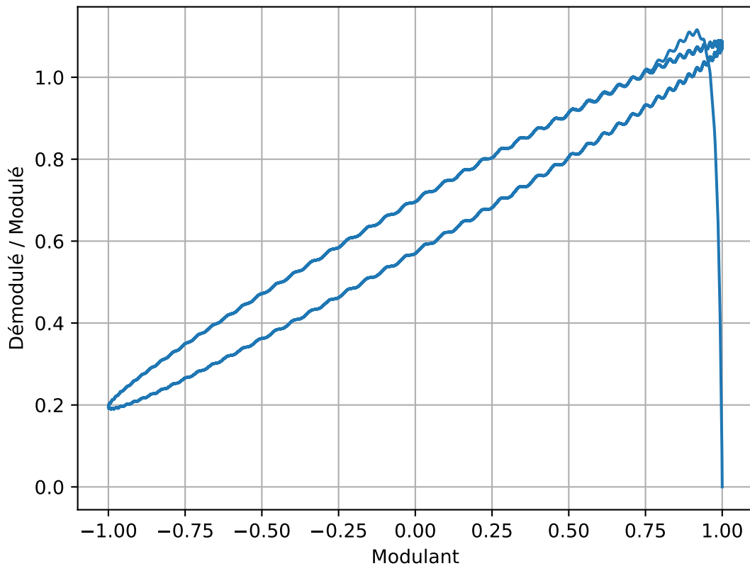
A3 — X-Y : modulant vs démodulé (crête)
