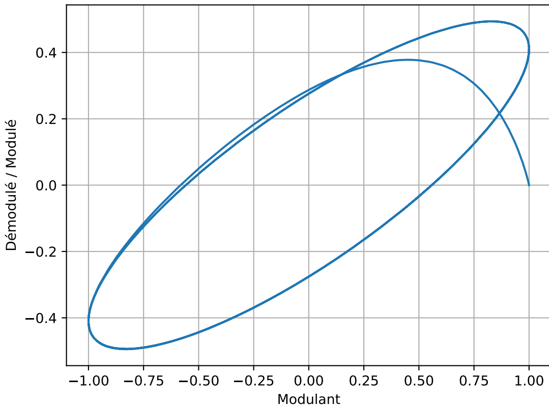
DSB-SC — X-Y : modulant vs démodulé (cohérent)
