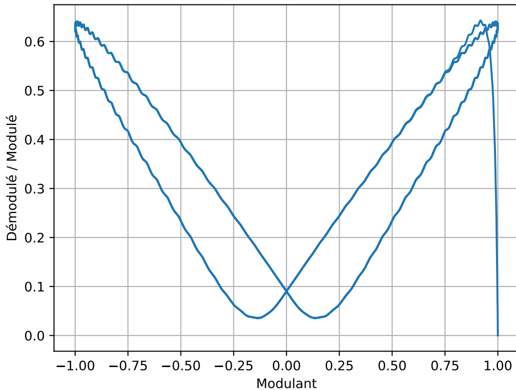
DSB-SC — X-Y : modulant vs démodulé (crête)
