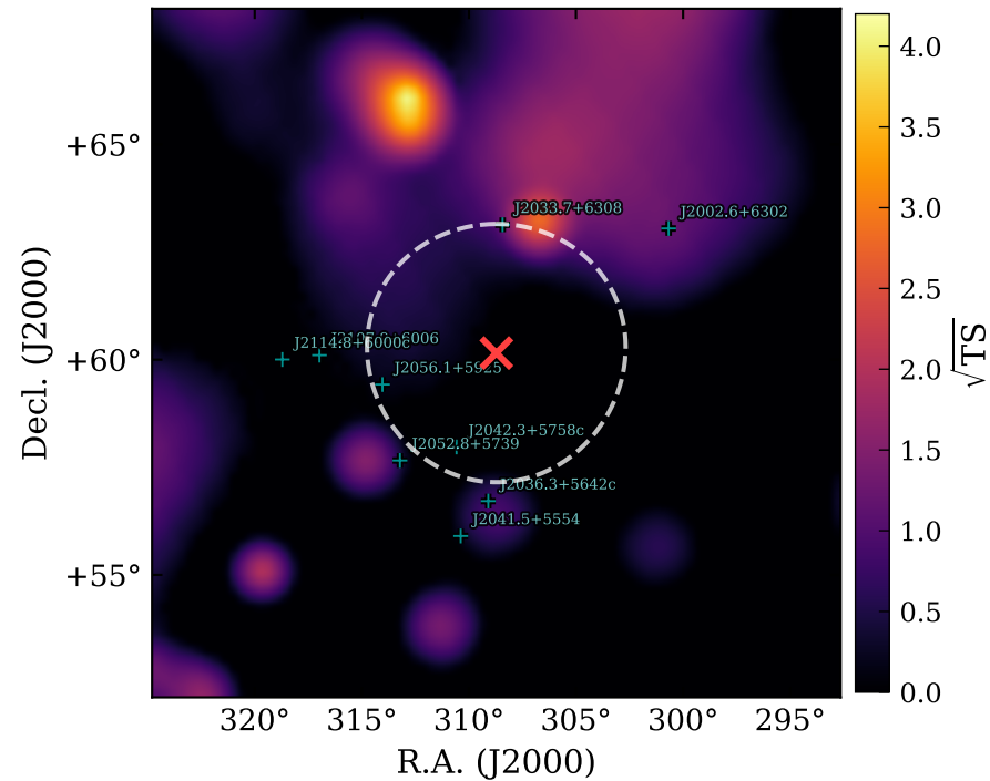
\sqrt{\text{TS}} (no GRB200423A)
