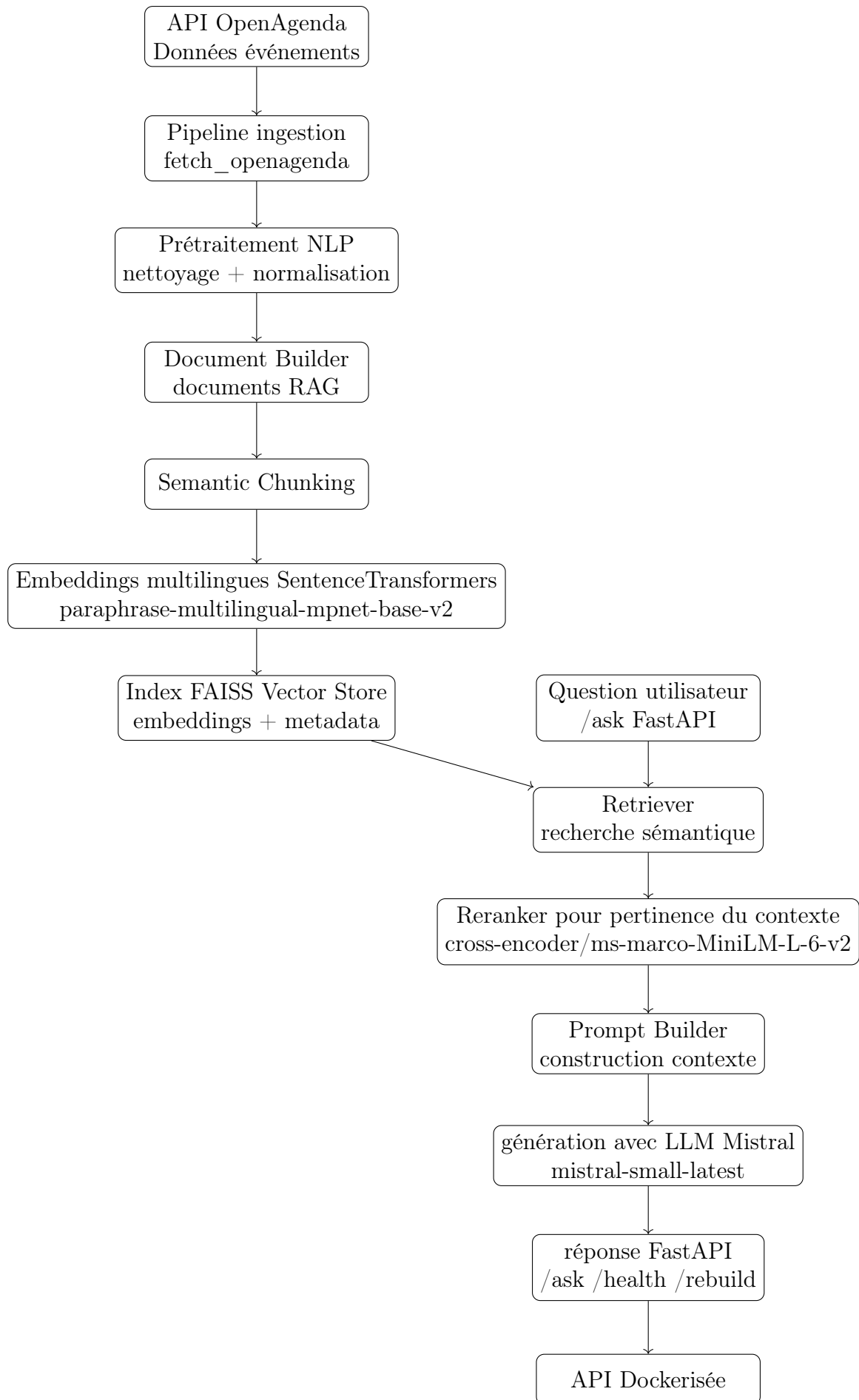
FIGURE 2.1 – Architecture globale du système RAG
