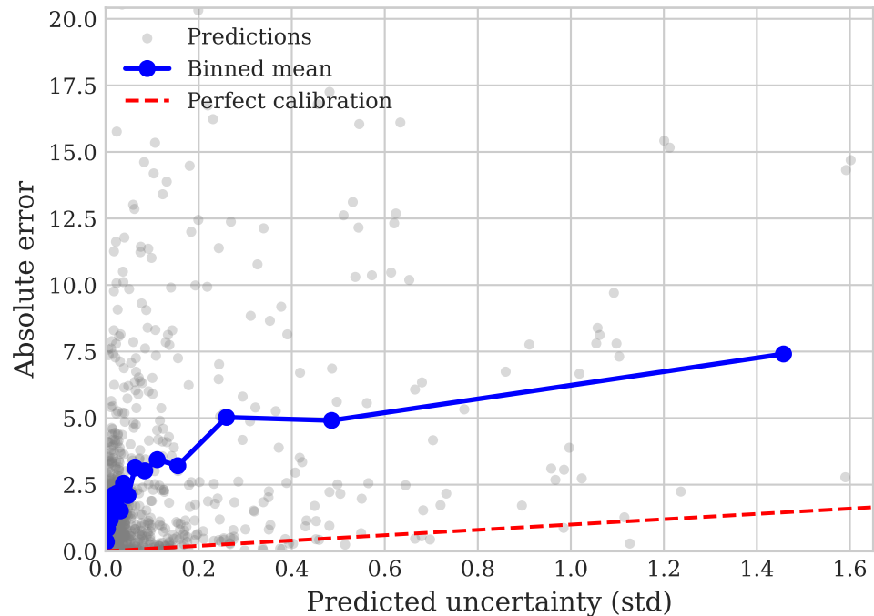
(a) Uncertainty vs. actual error
