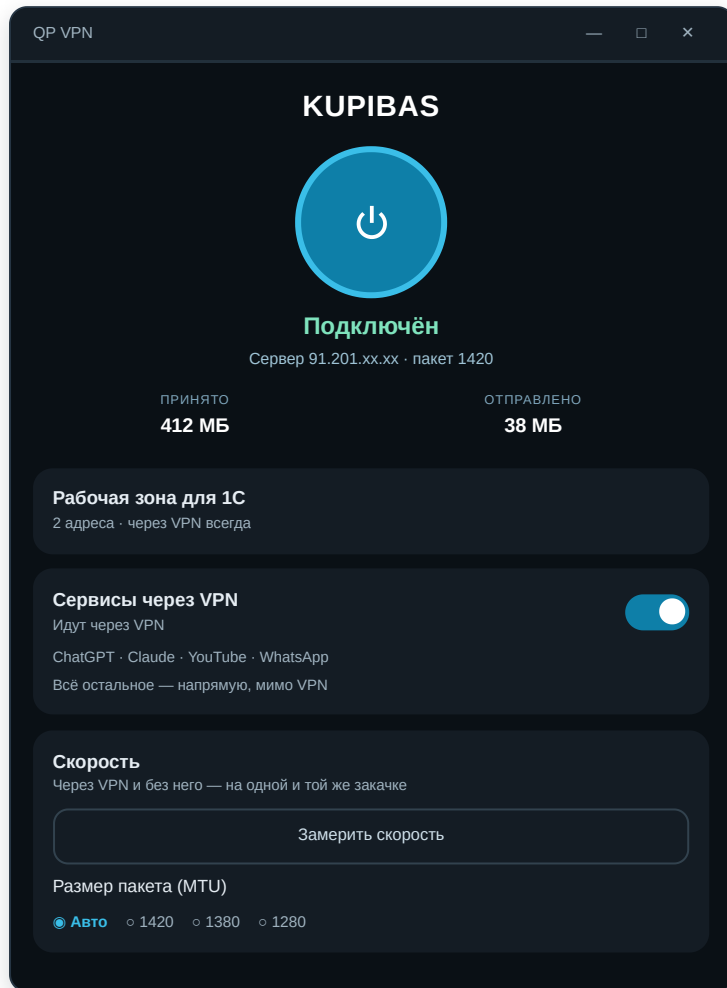
Главное окно
