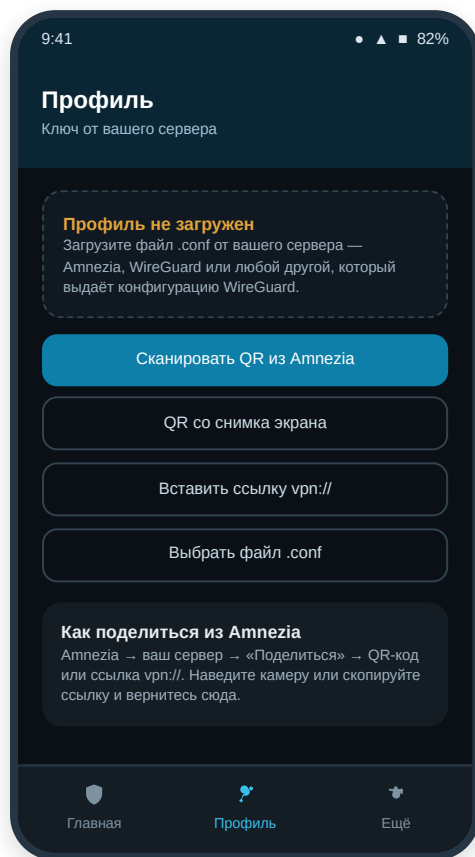
Вкладка «Профиль»
