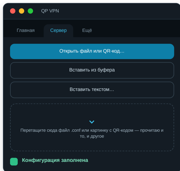
Вкладка «Сервер»
