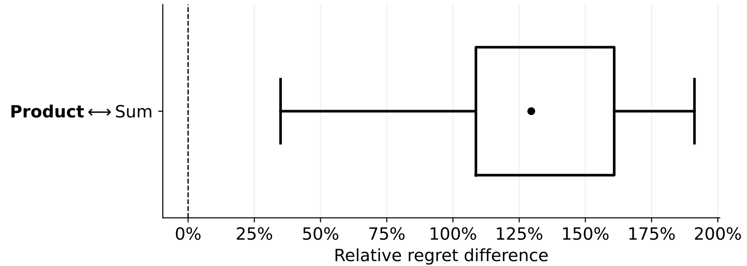
Svhn
