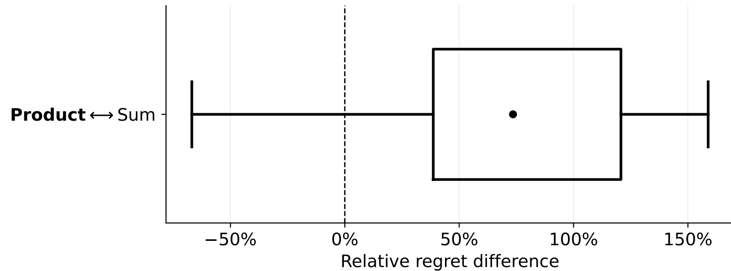
Cifar10
