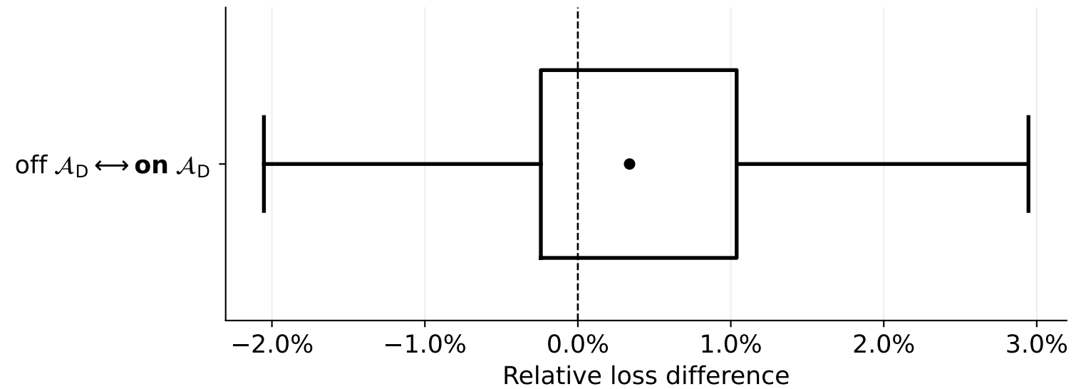
Cifar10
