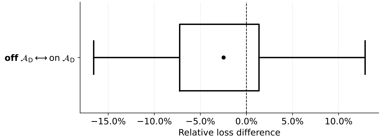
Svhn
