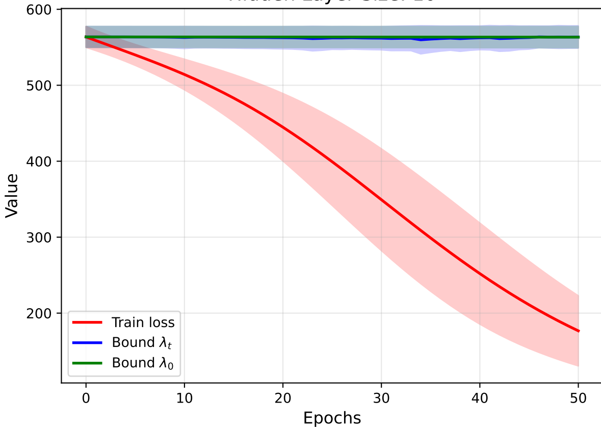
Hidden Layer Size: 10
