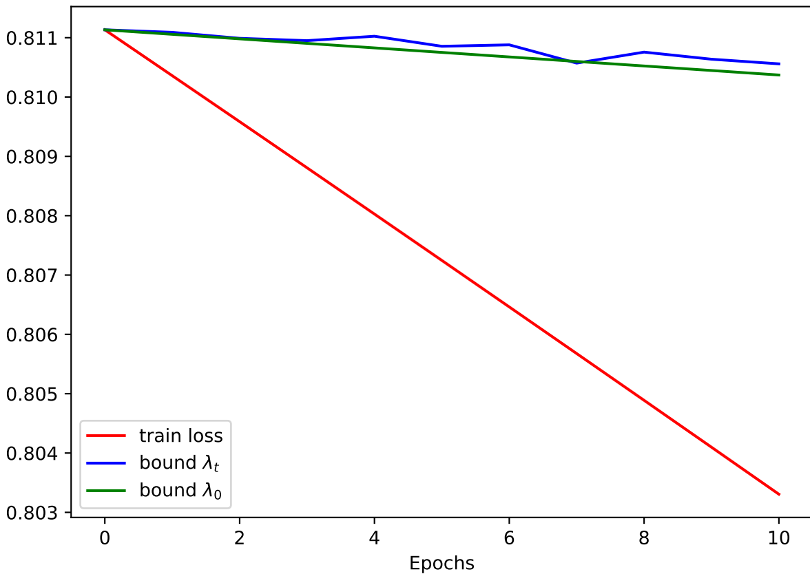
Hidden size : 1000
