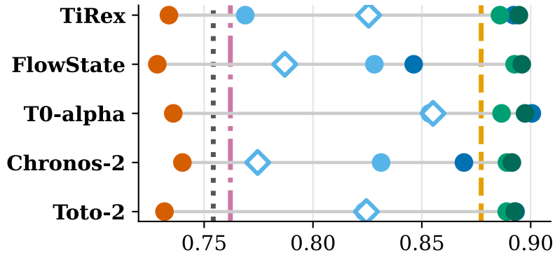
VUS-ROC
