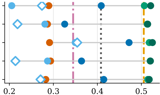
VUS-PR
