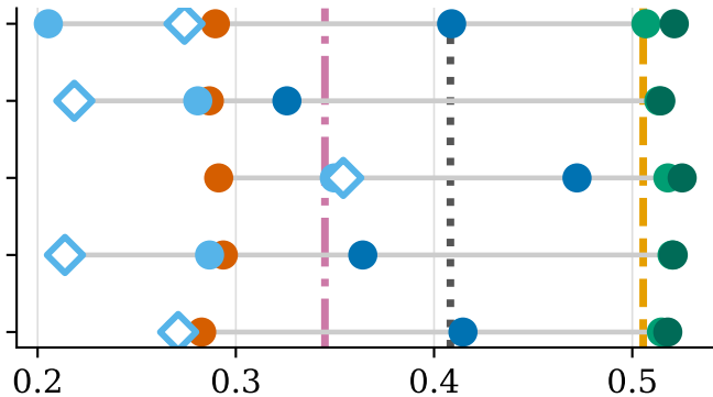
VUS-PR
