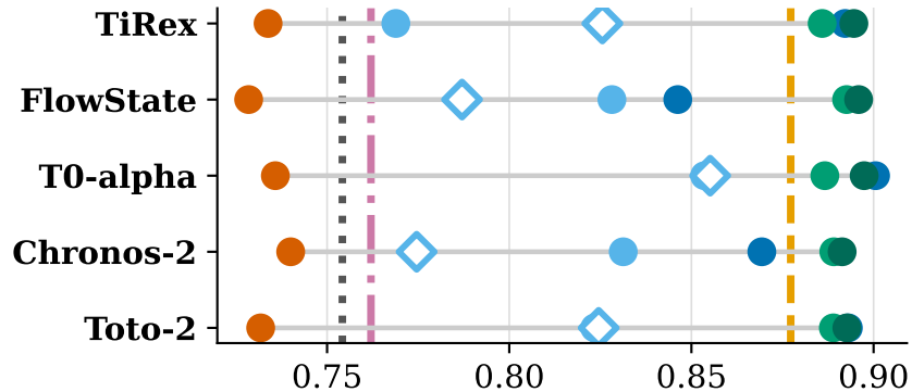
VUS-ROC
