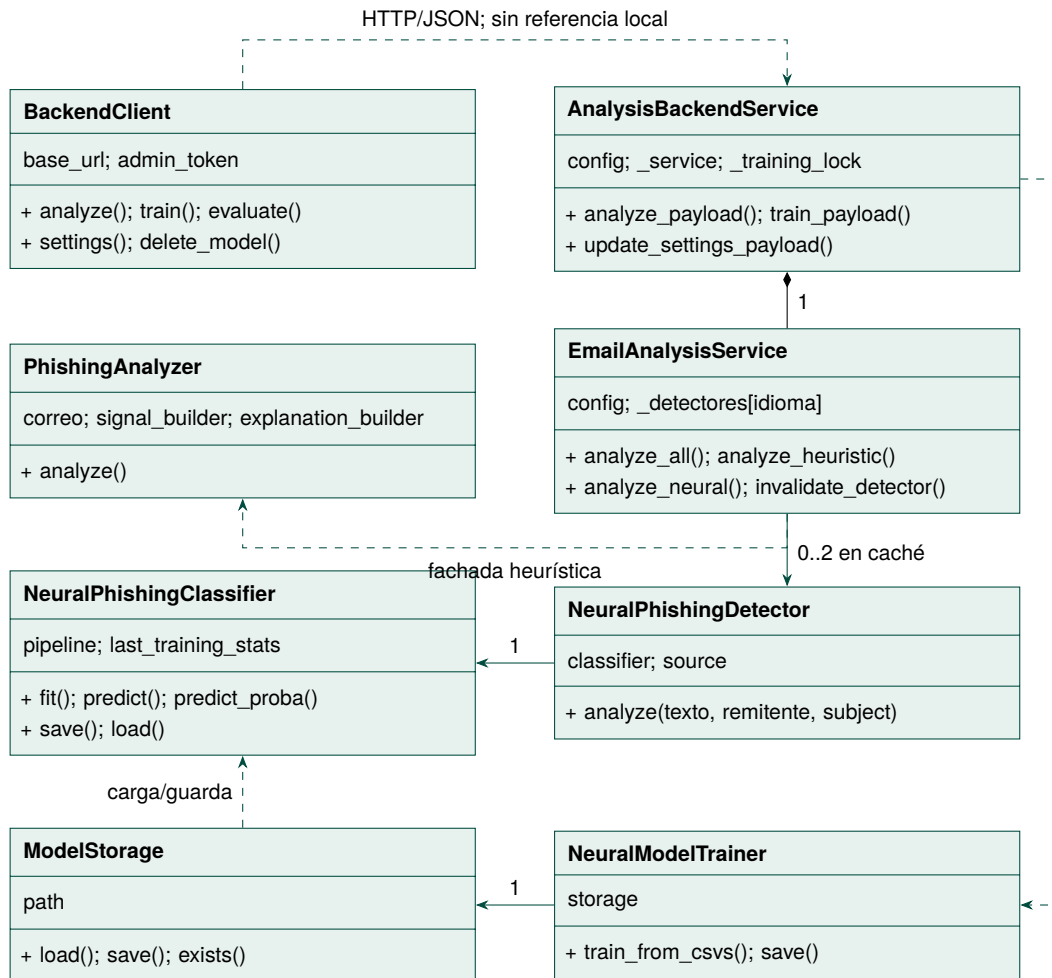
Figura 5.4: Clases principales y relaciones del análisis y aprendizaje. Rombo lleno: composición; línea continua: asociación; línea discontinua: dependencia. La relación entre cliente y servicio atraviesa la API. Fuente: elaboración propia.
