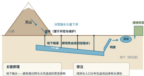
坎儿井结构与输水原理（剖面示意）
