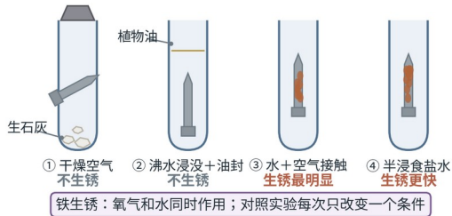
铁钉锈蚀条件的对比实验
