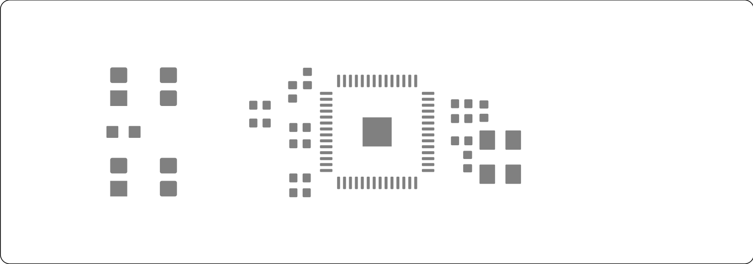
Top Paste (Scale 4:1)
