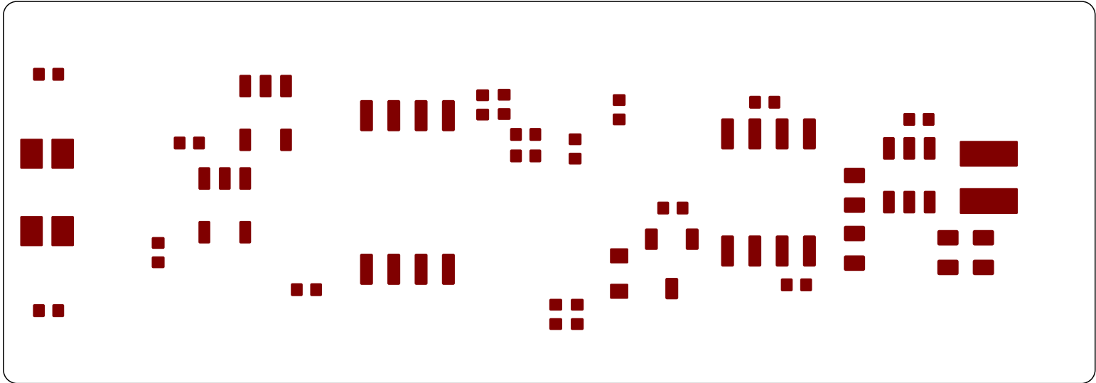
Bottom Paste (Scale 4:1)
