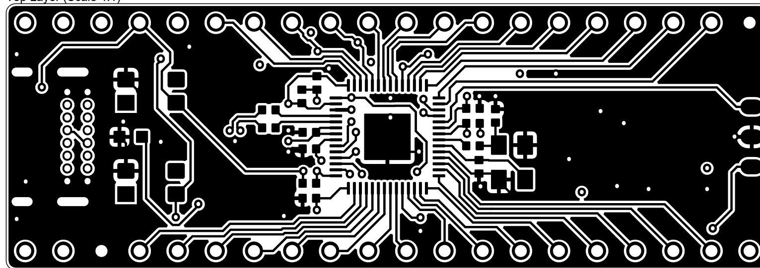
Top Layer (Scale 4:1)
