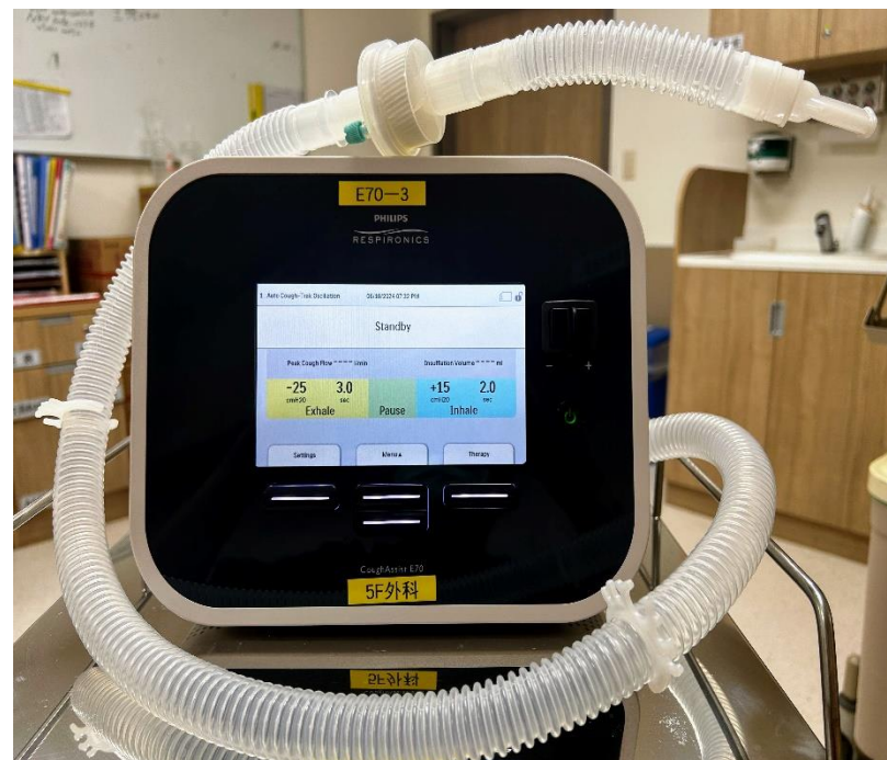
圖二：Cough Assist E70 管路組裝
