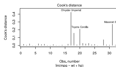
(d) Cook's distance
