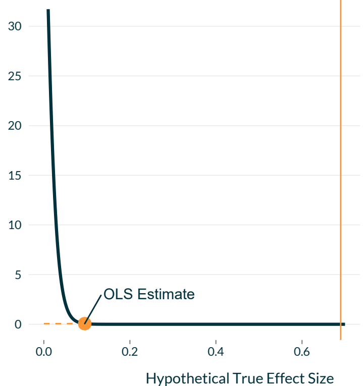
Type-S Error (%)
