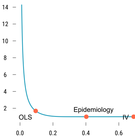
Type-M Error
