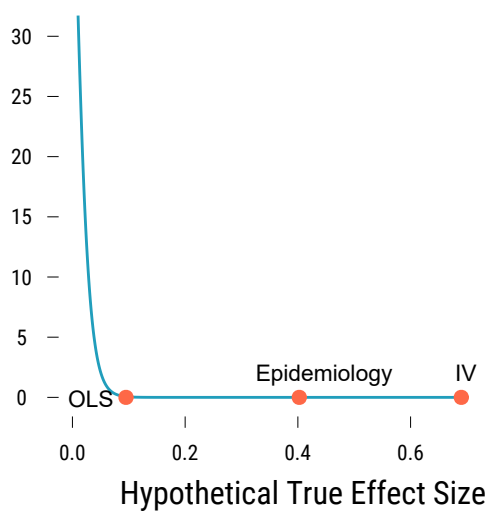
Type-S Error (%)
