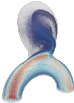
PI-MGN
