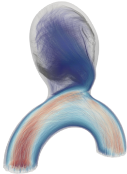
MGN
