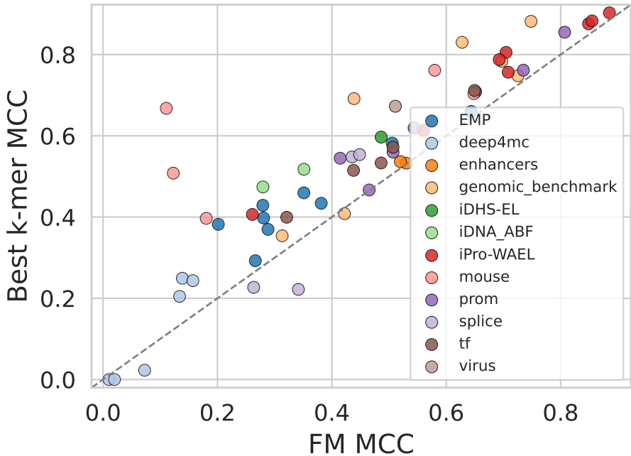
HyenaDNA-160k
