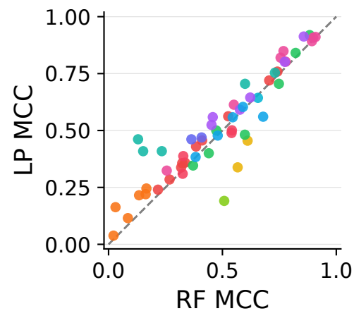
RF MCC Caduceus
