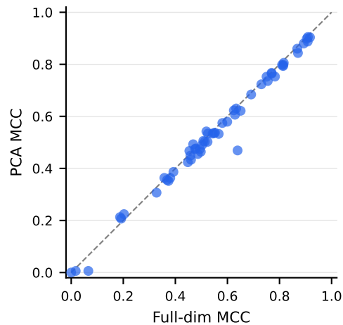
NTv3 med delta = -0.011
