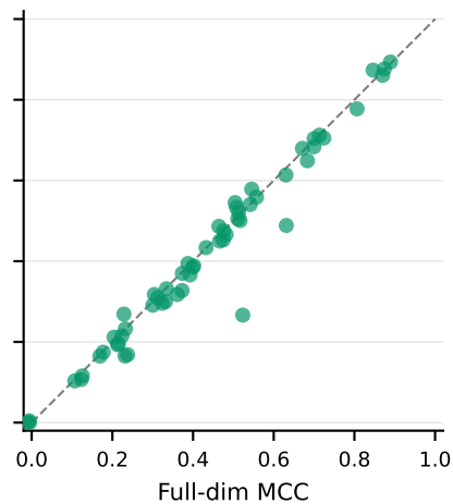
DNABERT-2 med delta = -0.004
