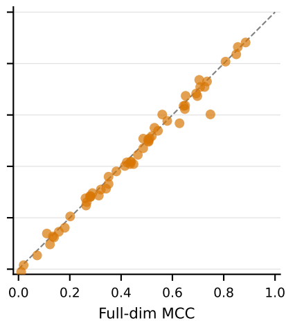
HyenaDNA med delta = -0.008
