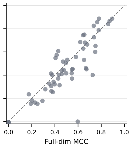
k-mer k=6 med delta = -0.025
